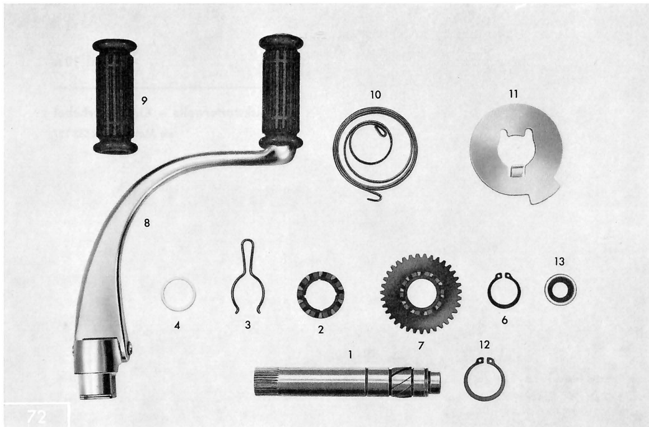
Tafel 10 a Kickstarterwelle – Kickstarterhebel
