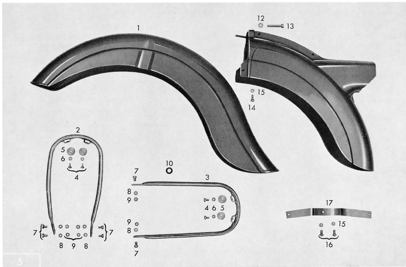
Tafel 14 Schutzbleche
