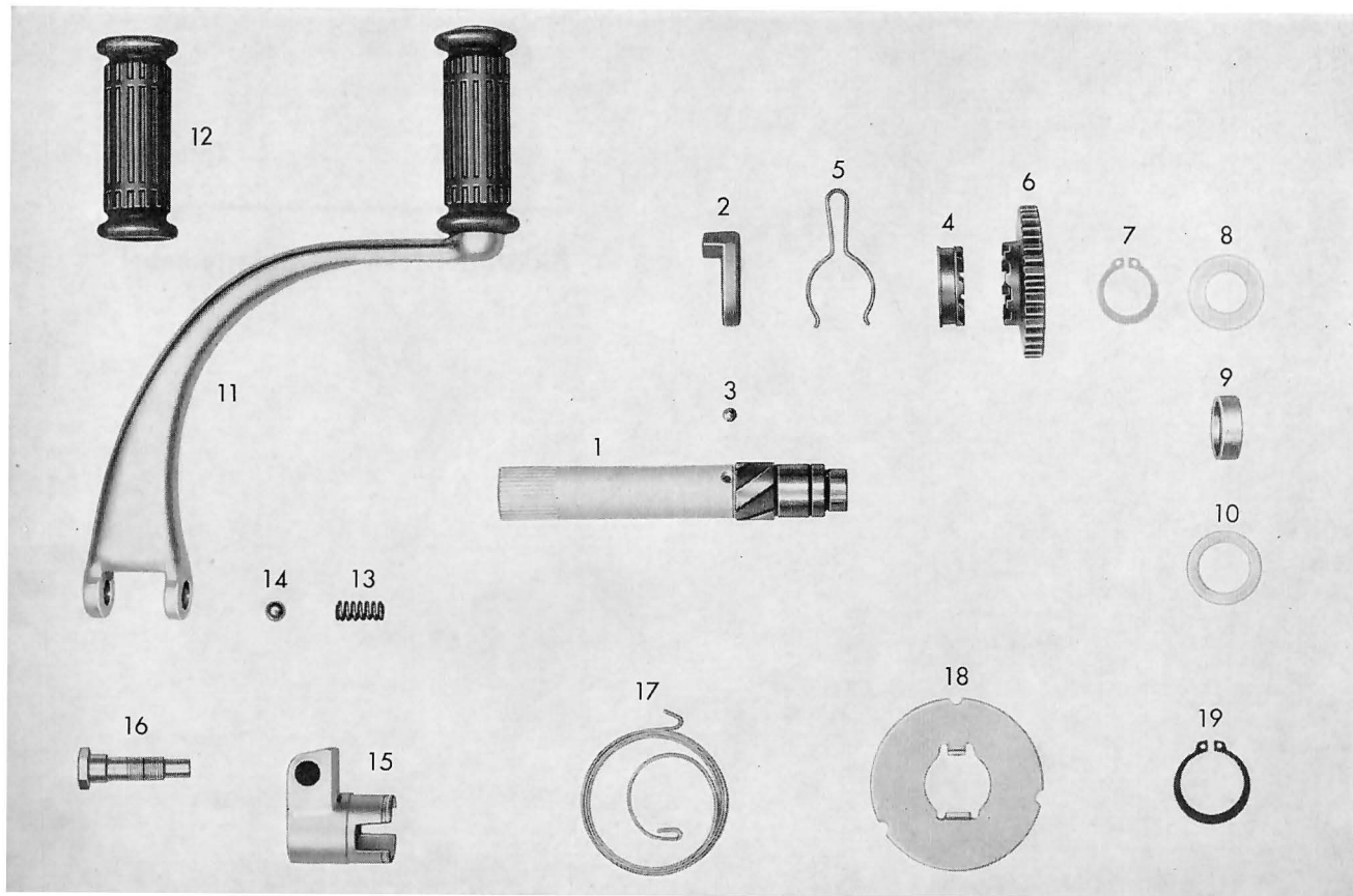
Tafel 10 Kickstarterwelle – Kickstarterhebel
