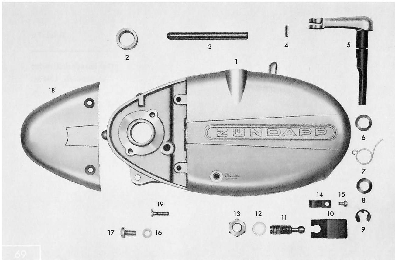
Tafel 4 a Gehäusedeckel rechts
