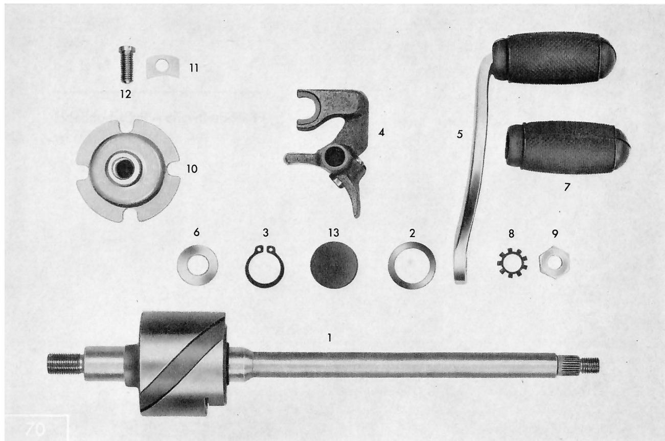
Tafel 9 a Fußschaltwelle – Fußschalthebel
