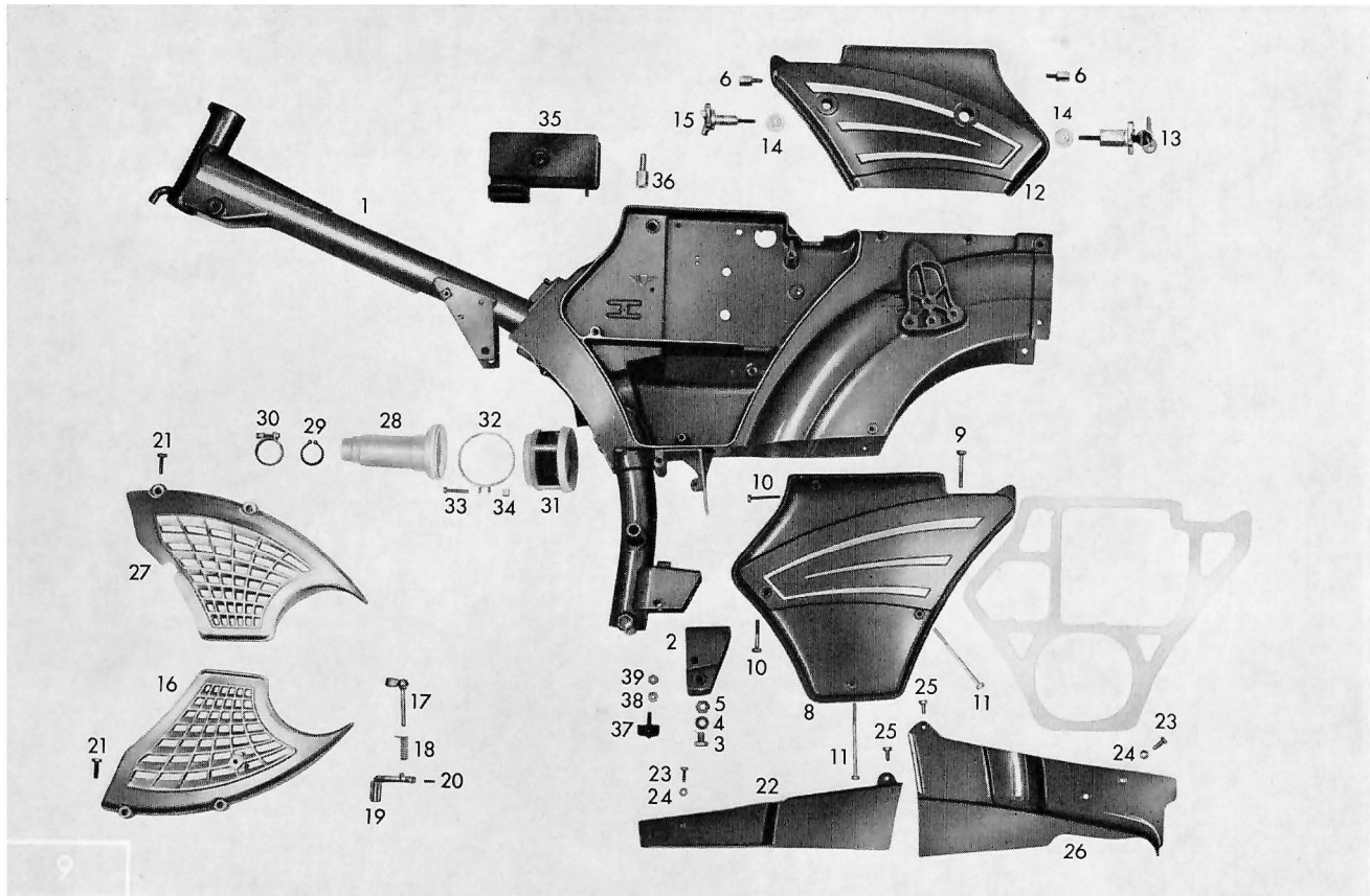
Tafel 1 Rahmen
