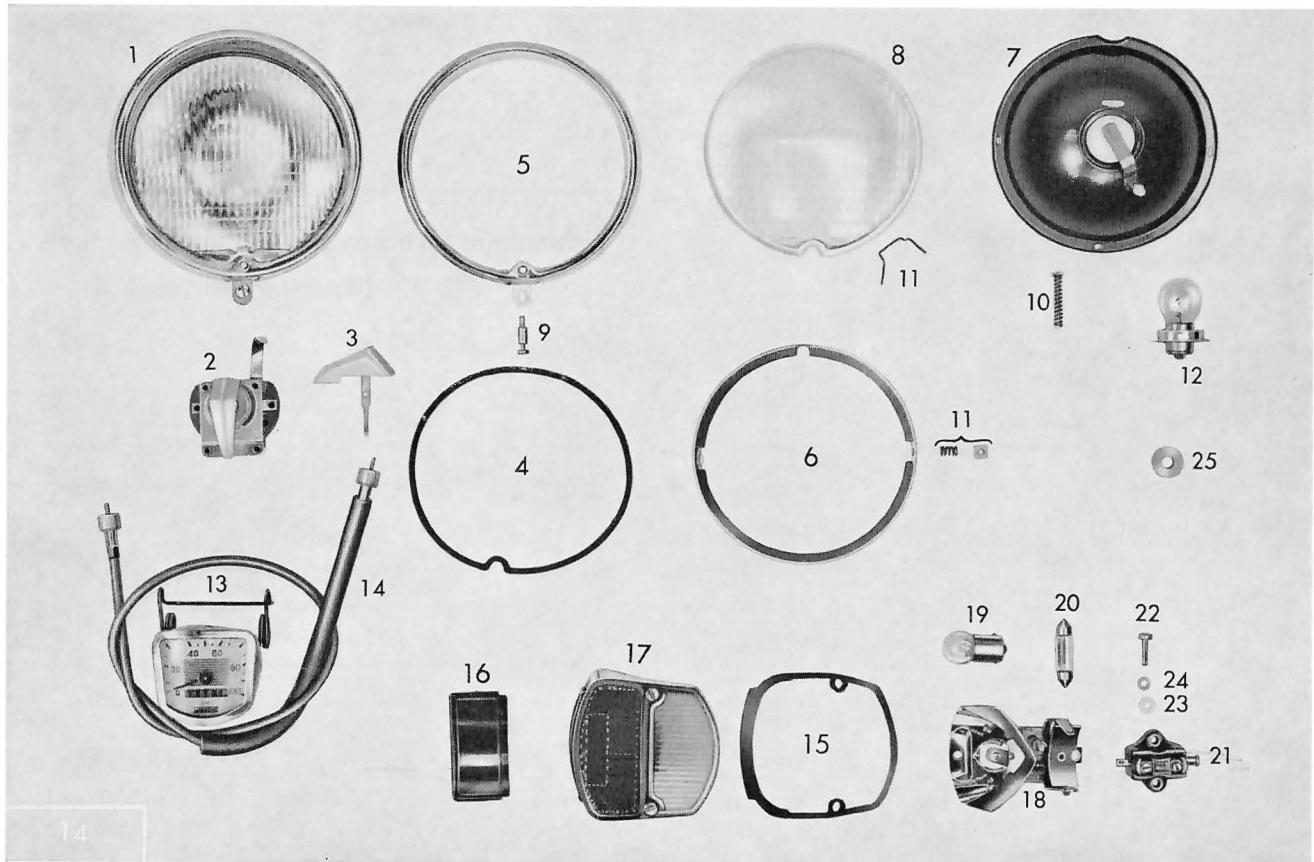
Tafel 9 Lichtanlage – Tachometer – Stopplicht (dauerabgeblendet)
