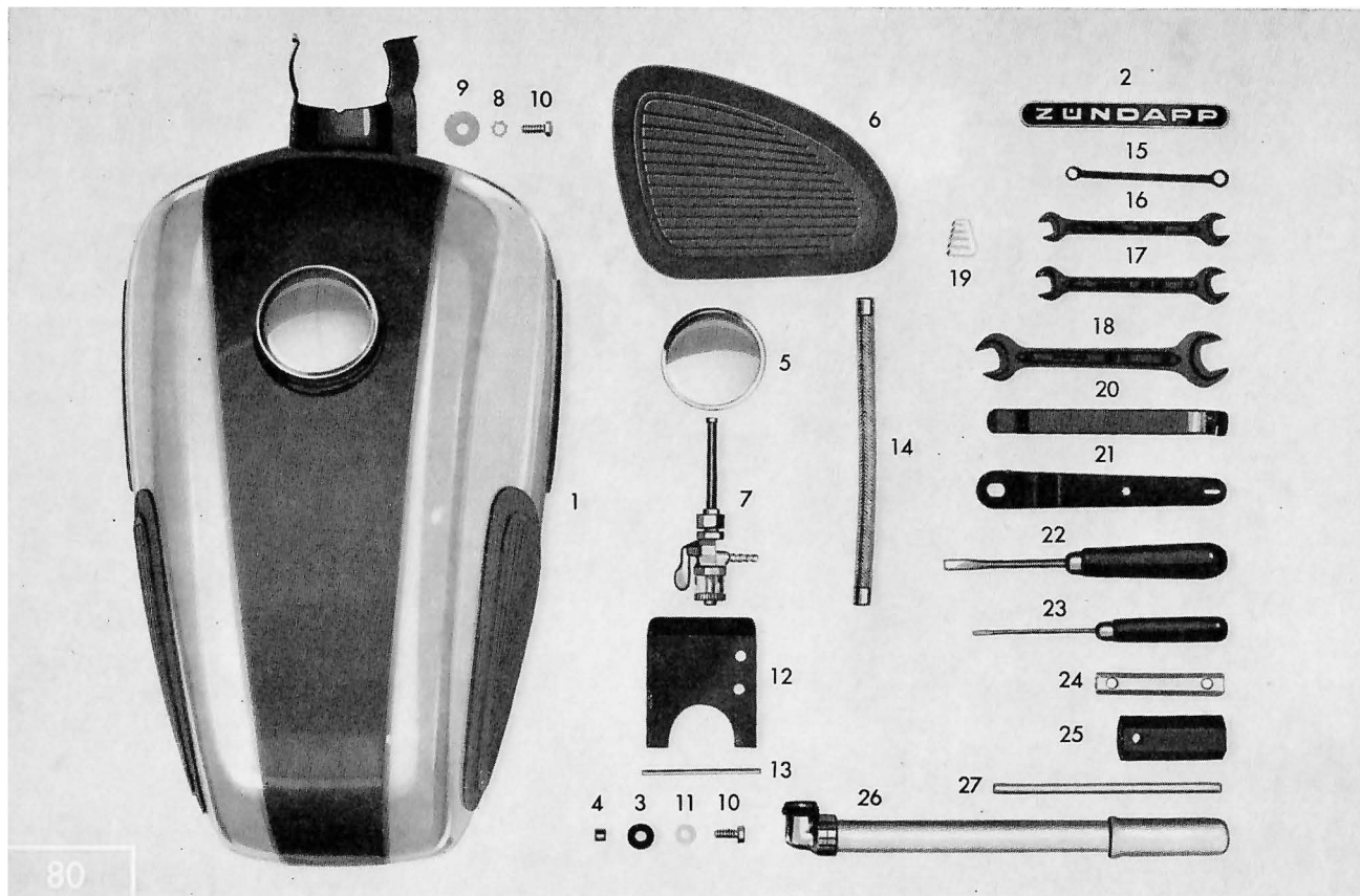
Tafel 15 a Kraftstoffbehälter – Werkzeuge
