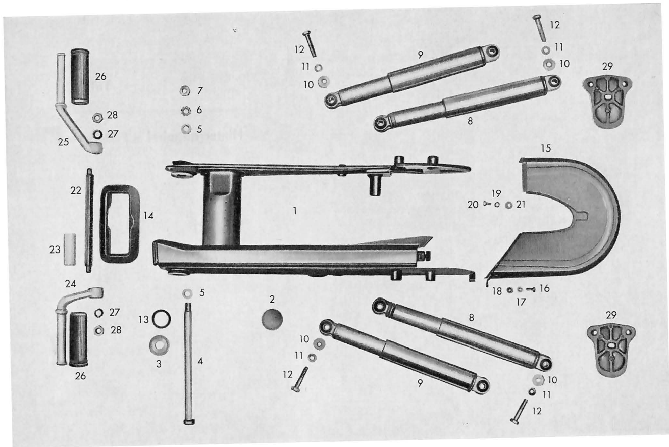
Tafel 4 Hinterradgabel – Federbein
