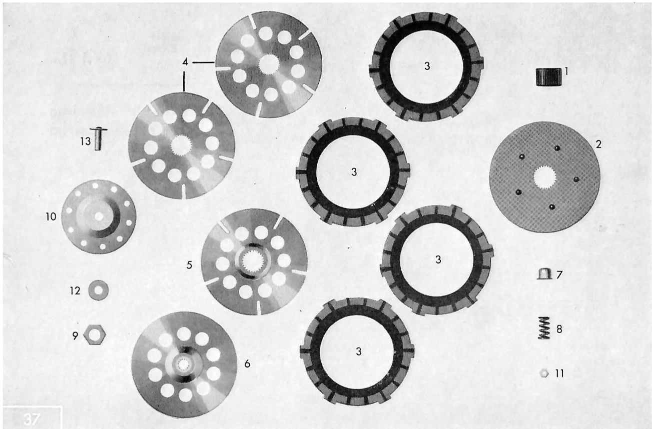
Tafel 11 a Kupplung
