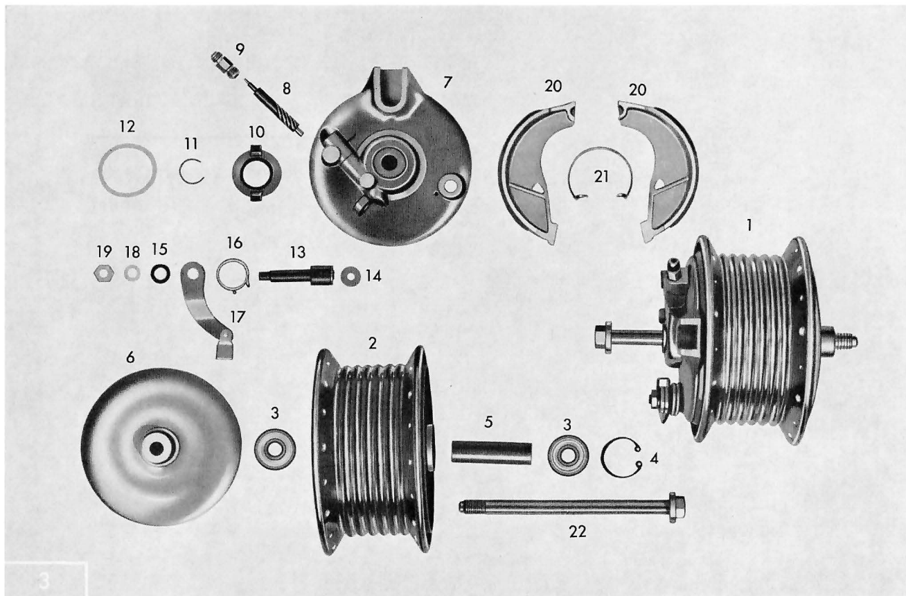
Tafel 5 Vorderes Laufrad – Vorderradnabe 21" Räder
