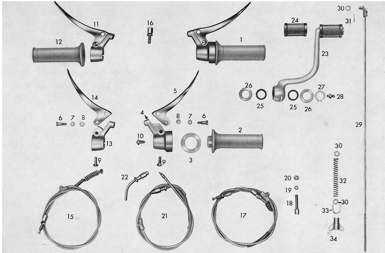
Tafel 12 Schalt-, Betätigungshebel – Züge (Fußschaltung)
