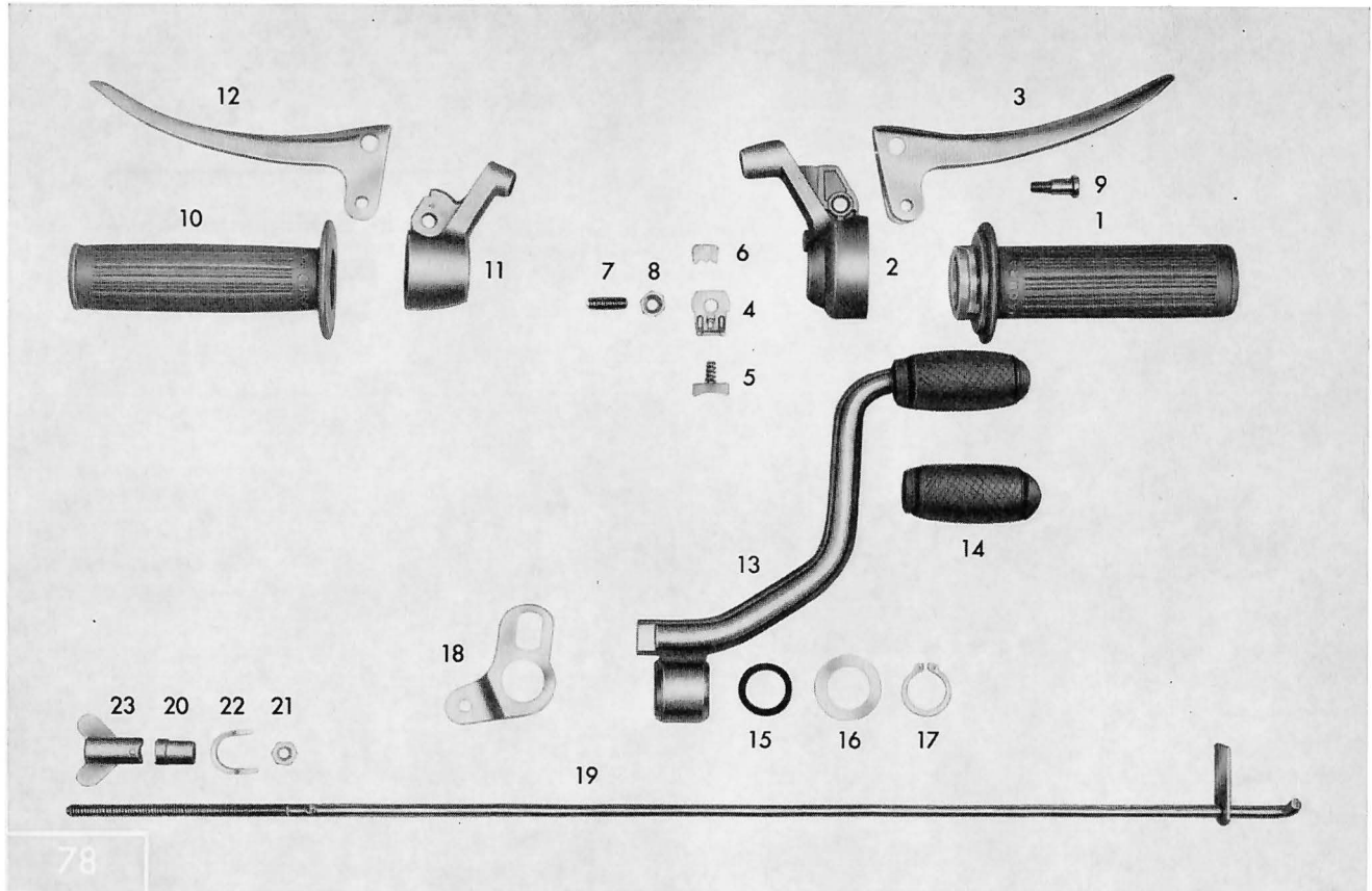
Tafel 12 a Schalt-, Betätigungshebel – Züge (Fußschaltung)
