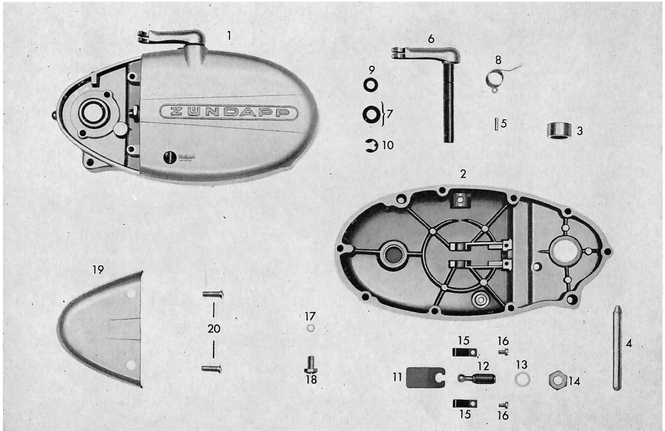
Tafel 4 Gehäusedeckel rechts
