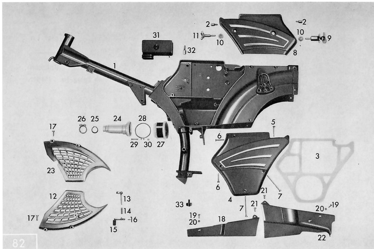
Tafel 1 a Rahmen
