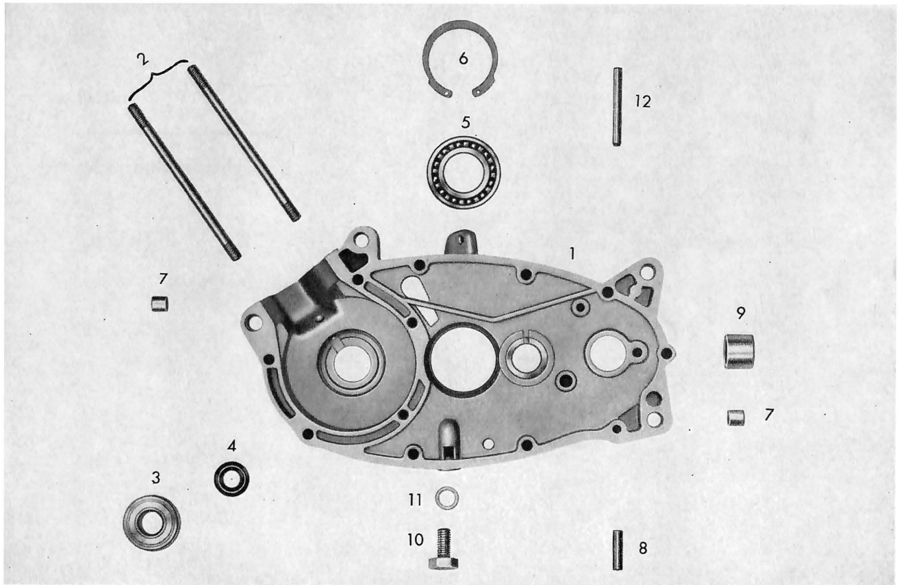
Tafel 1 Gehäusehälfte rechts
