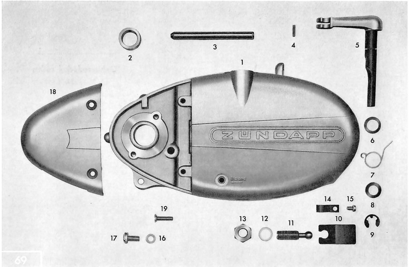
Tafel 4 a Gehäusedeckel rechts
