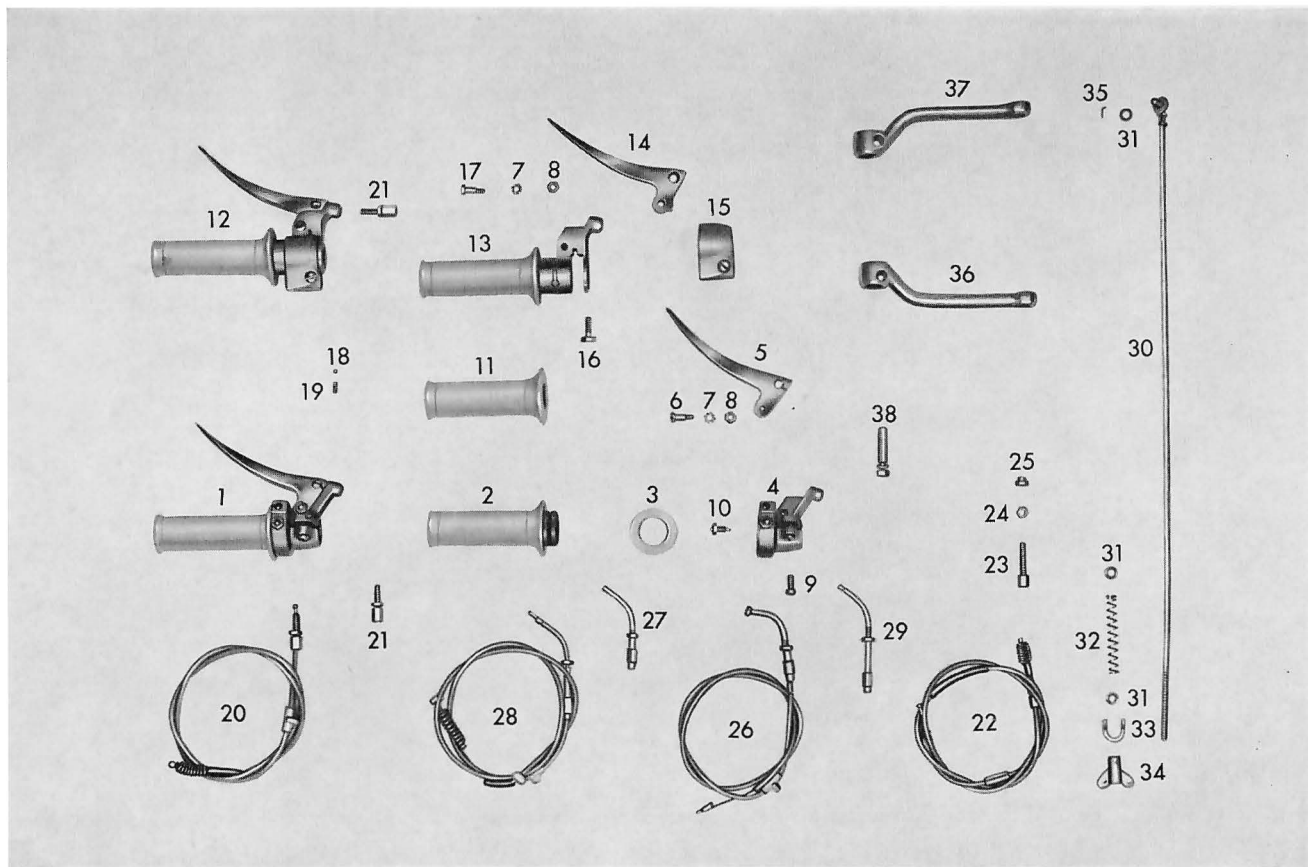
Tafel 13 Schalt-, Betätigungshebel – Züge (Handschtaltung)
