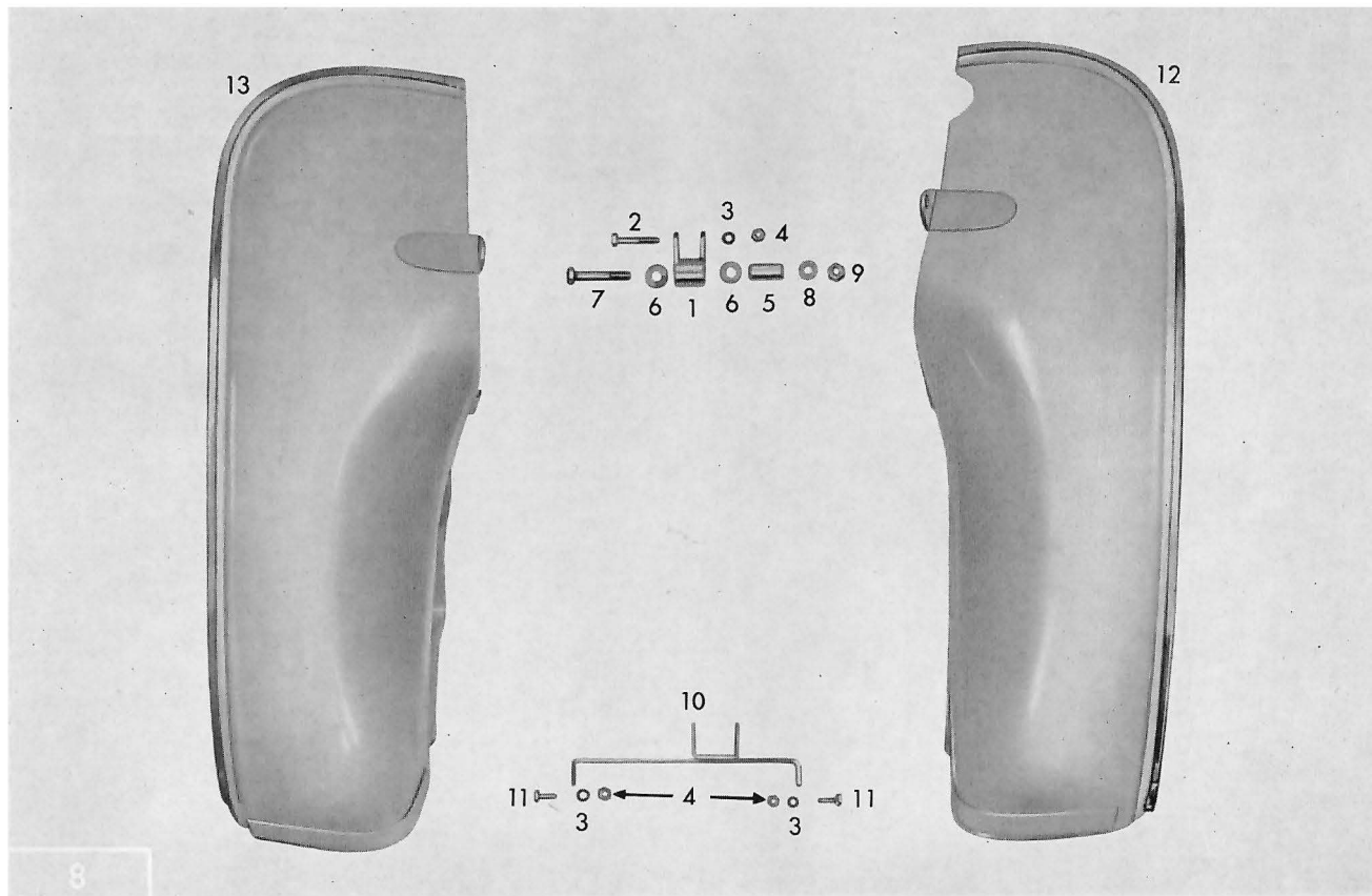
Tafel 18 Beinschild
