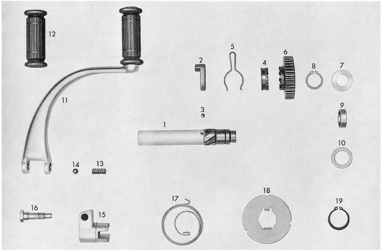
Tafel 10 Kickstarter – Kickstarterhebel
