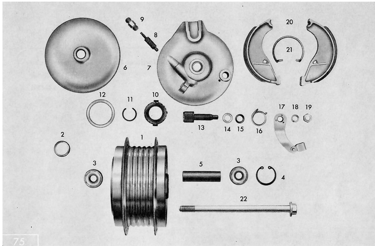
Tafel 5 a Vorderes Laufrad – Vorderradnabe 21" Räder
