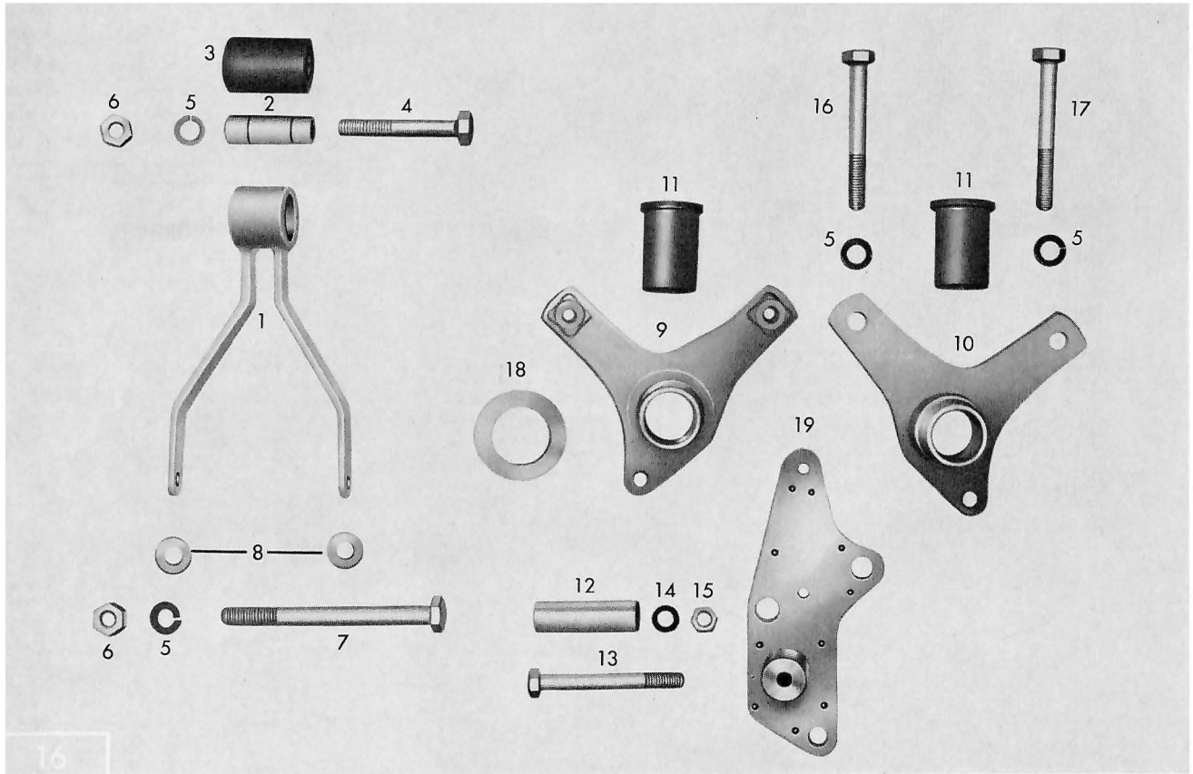
Tafel 2 Motoraufhängung
