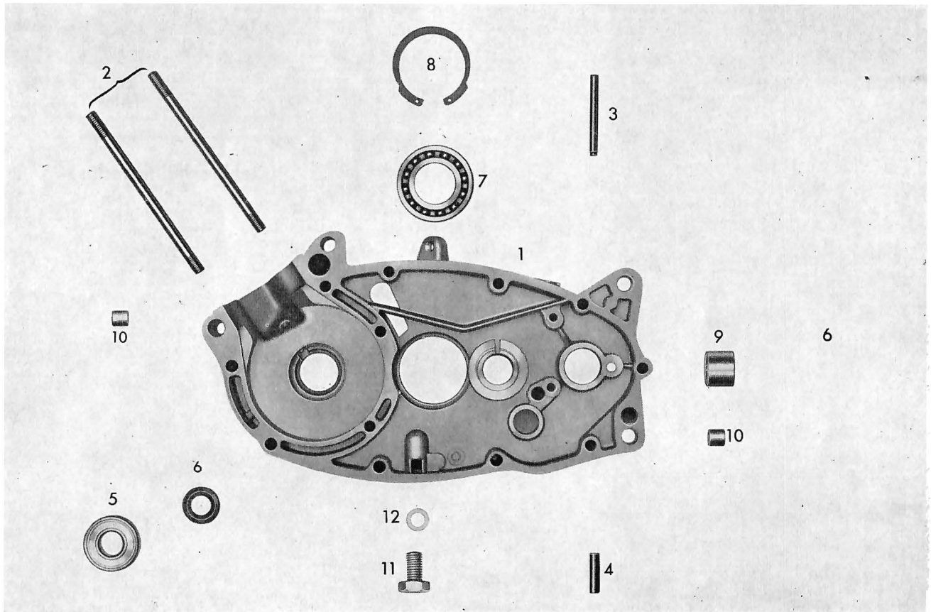
Tafel 1 Gehäusehälfte rechts
