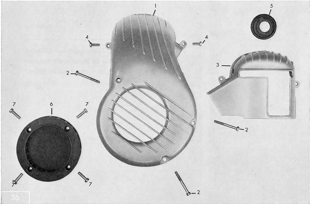
Tafel 3 a Lüftergehäuse – Lüfterrad (nur für Motoren mit Gebläse)
