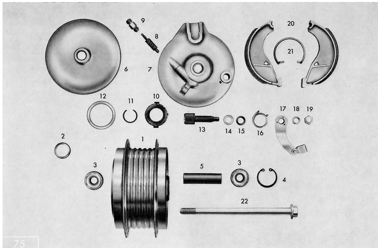
Tafel 6 a Vorderes Laufrad – Vorderradnabe 23" Räder
