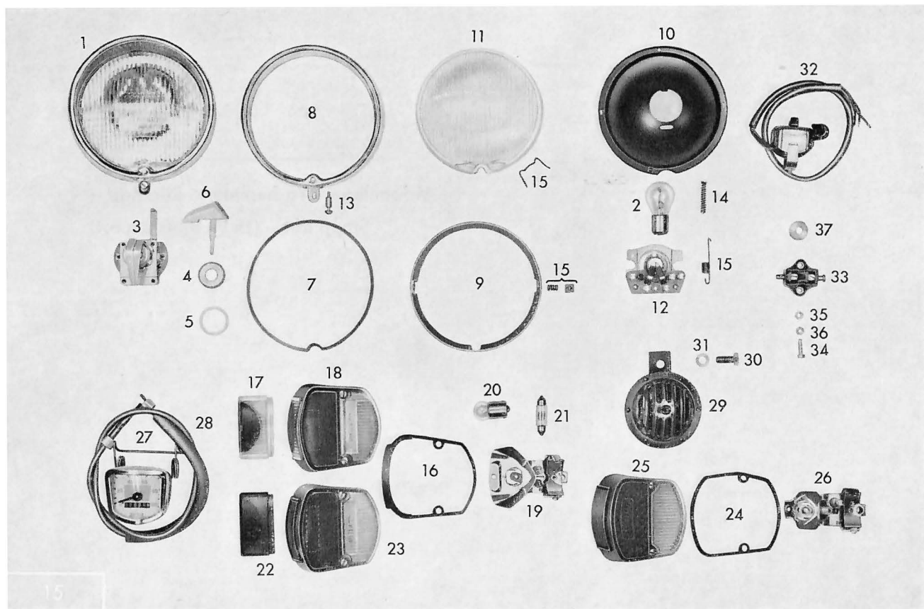
Tafel 11 Lichtanlage – Tachometer – Rücklicht – Stopplicht – (15 W Bilux Export)
