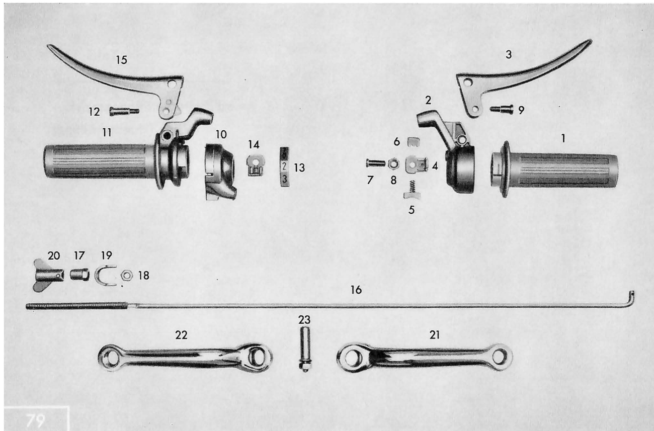
Tafel 13 a Schalt-, Betätigungshebel – Züge (Handschaltung)
