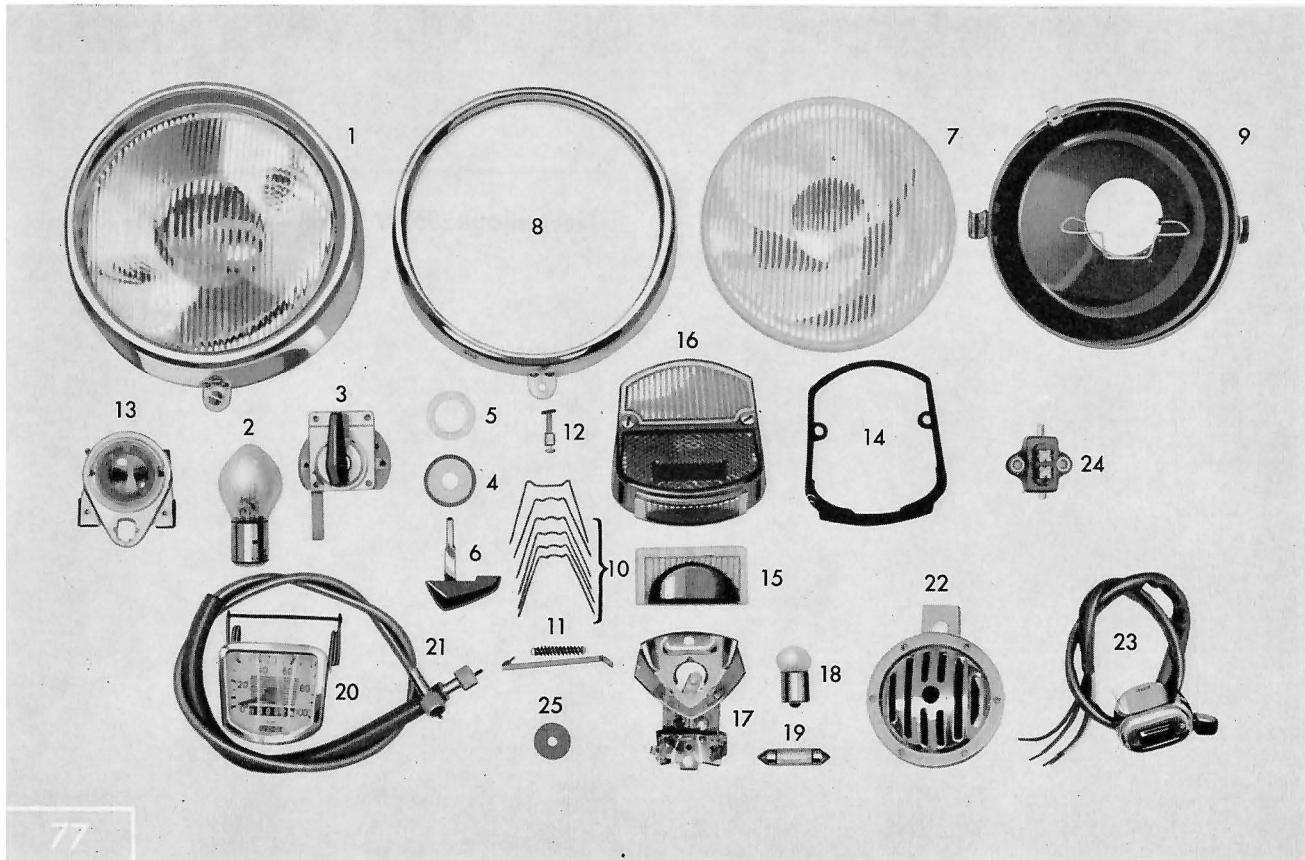
Tafel 10 a Lichtanlage (25 W Bilux) – Tachometer – Stopplicht
