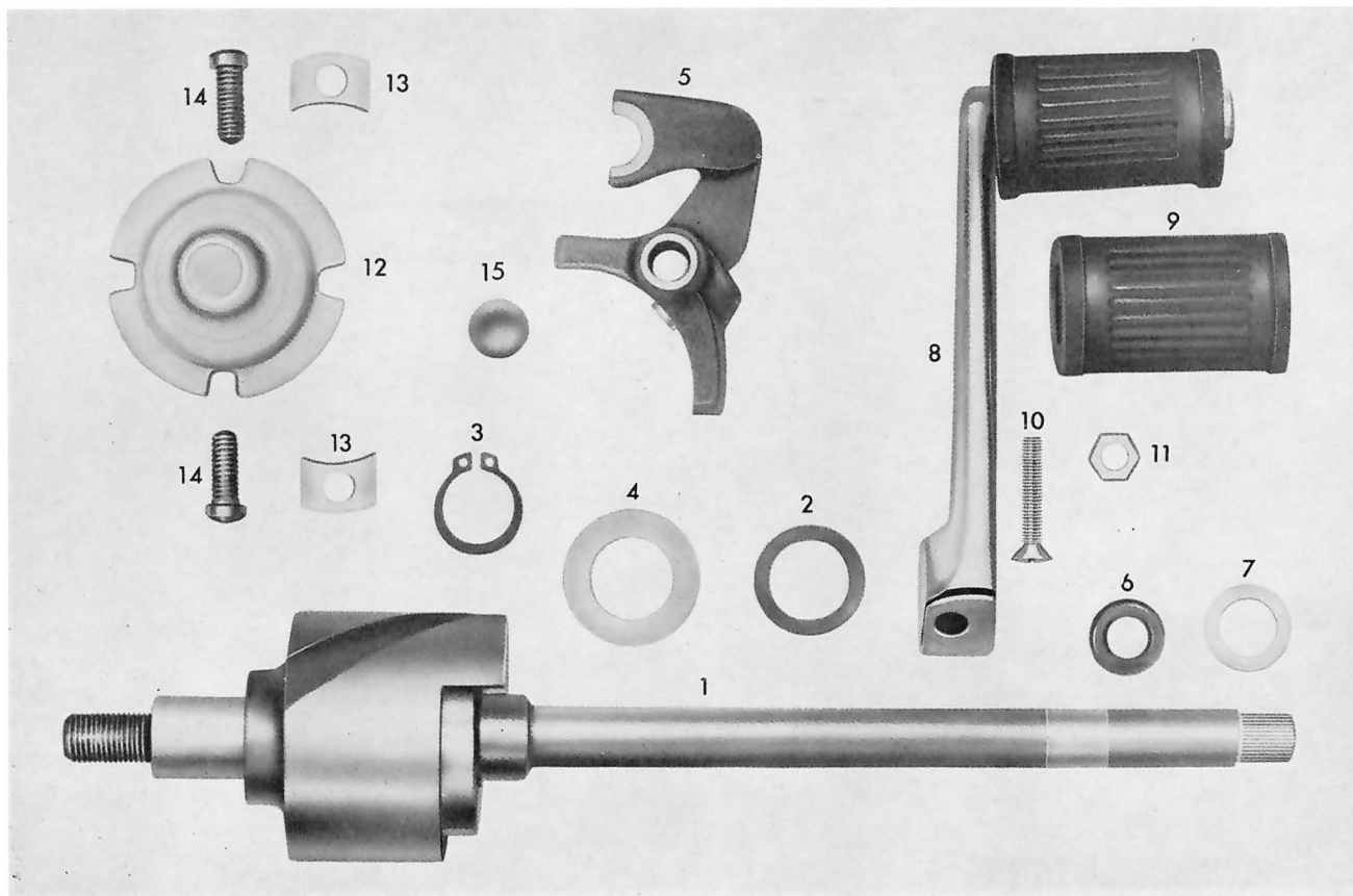
Tafel 9 Fußschaltwelle – Fußschalthebel
