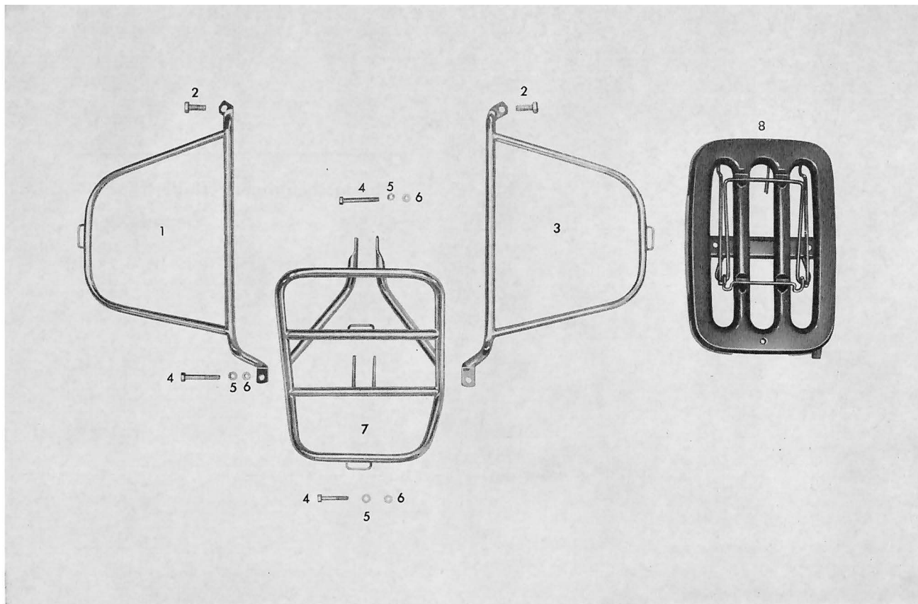
Tafel 17 Packtaschenträger – Kofferträger – Gepäckträger
