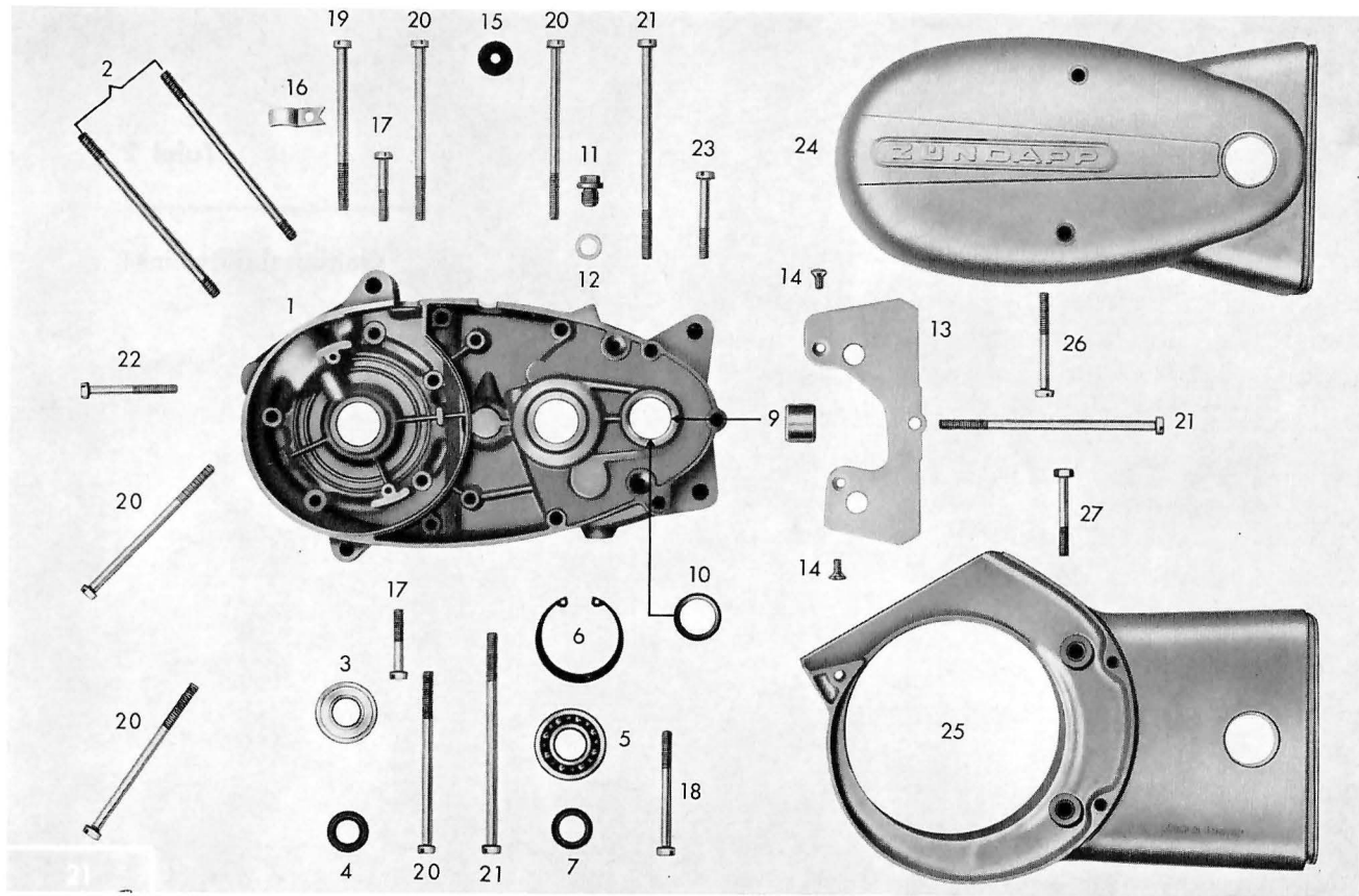
Tafel 2 Gehäusehälfte links
