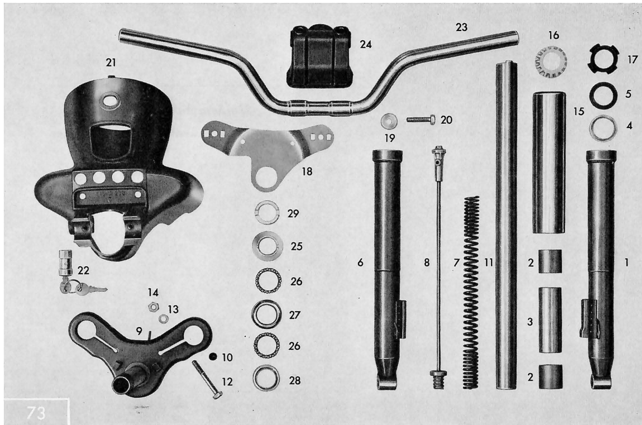
Tafel 3 a Vordergabel – Gabelgehäuse – Lenkungslager – Lenker
