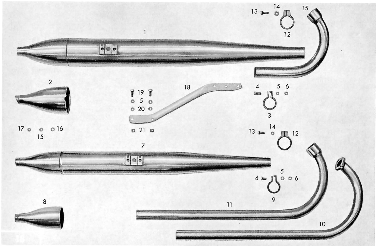
Tafel 13 Auspuff
