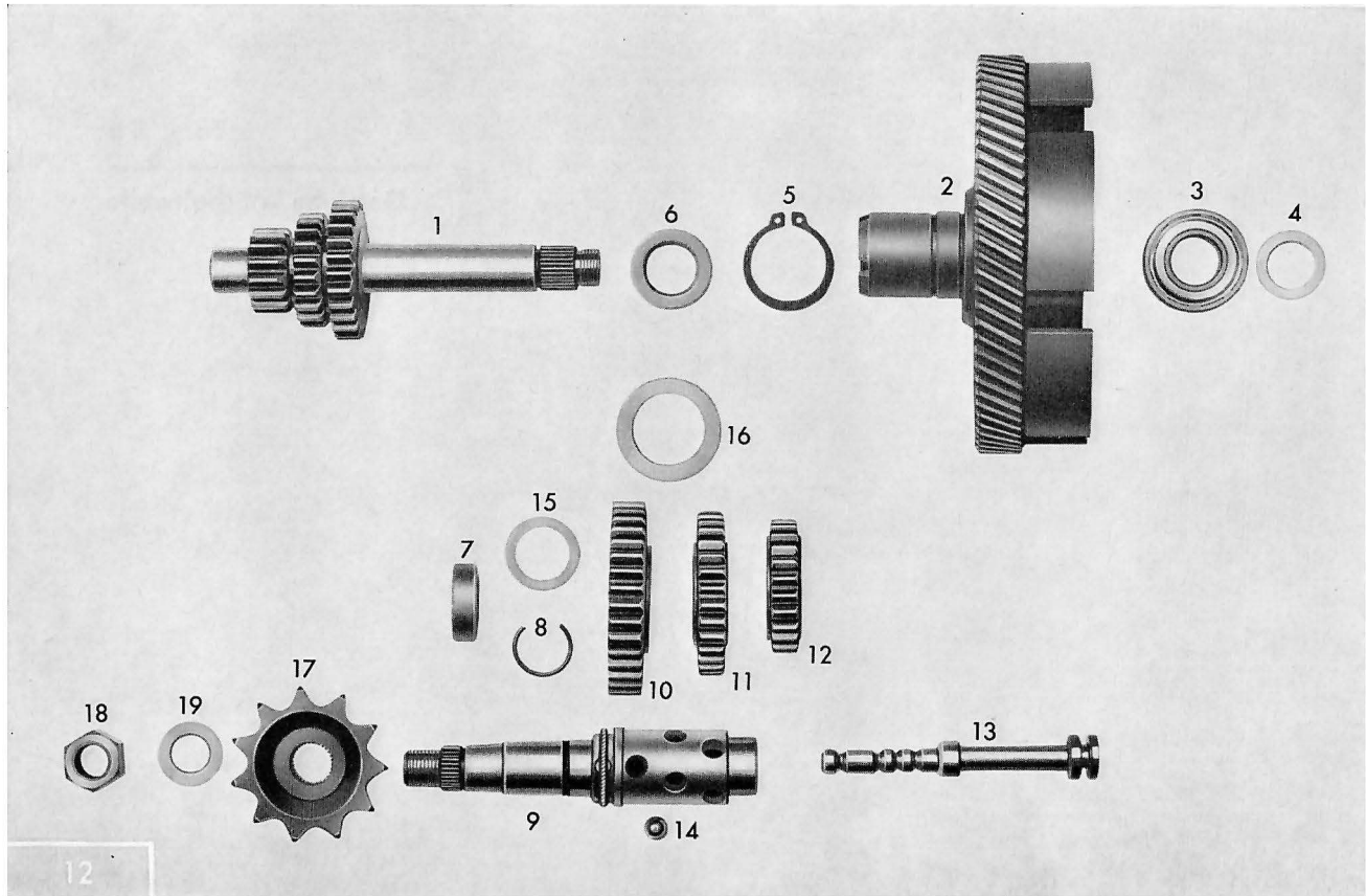
Tafel 8 a Getriebe – Schaltwelle
