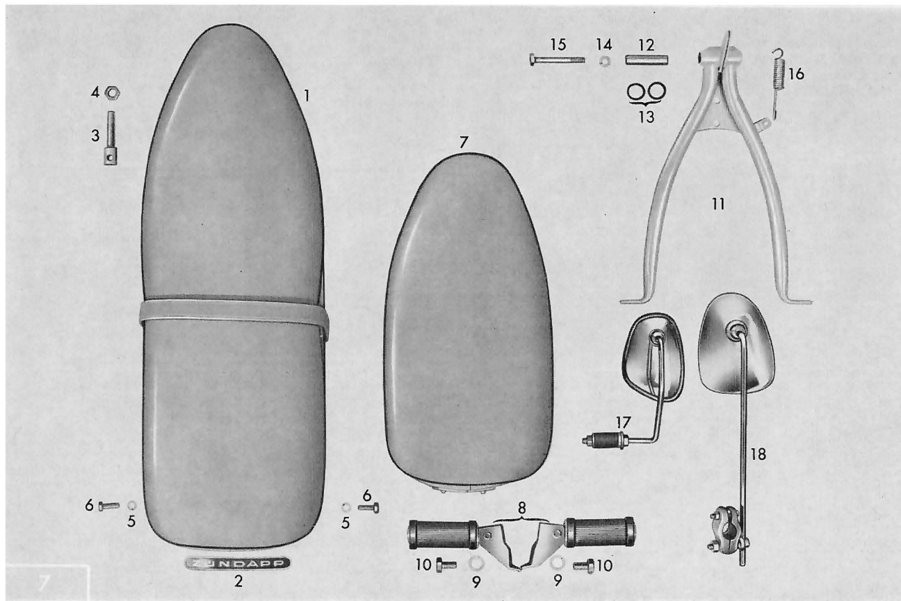
Tafel 16 Doppelsitzbank – Einzelsitzbank – Radständer
