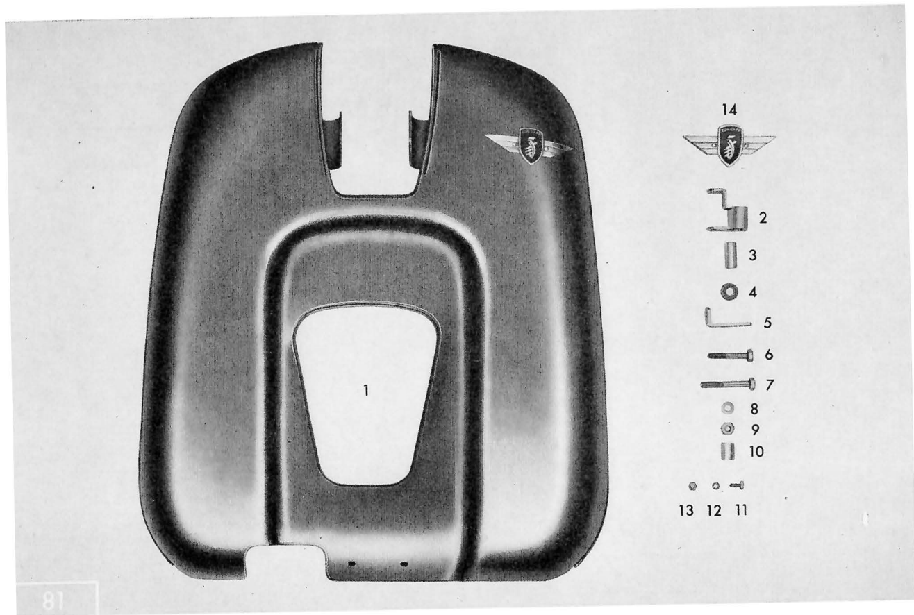
Tafel 18 a Beinschild
