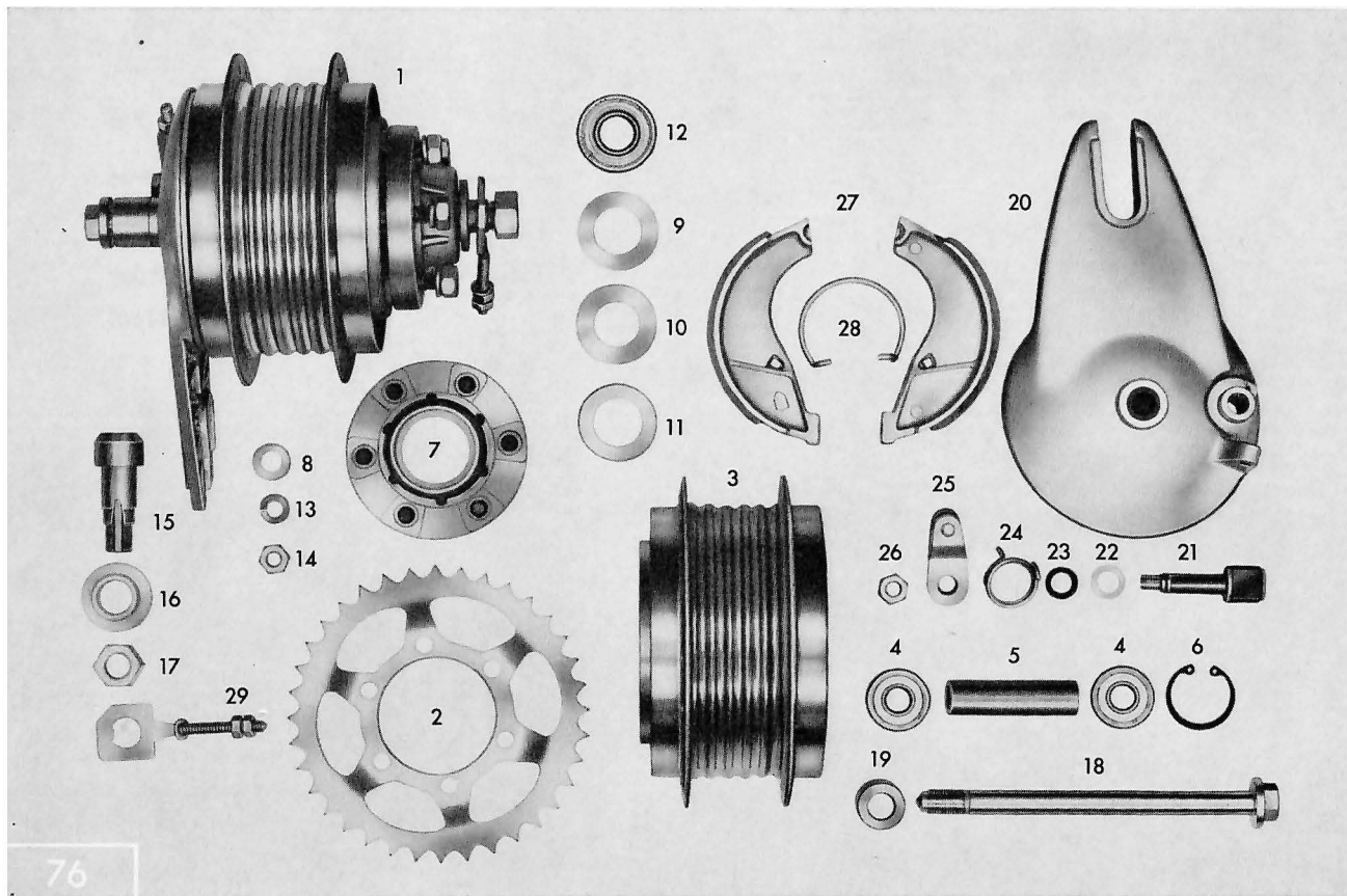
Tafel 7 a Hinteres Laufrad – Hinterradnabe 21" Räder
