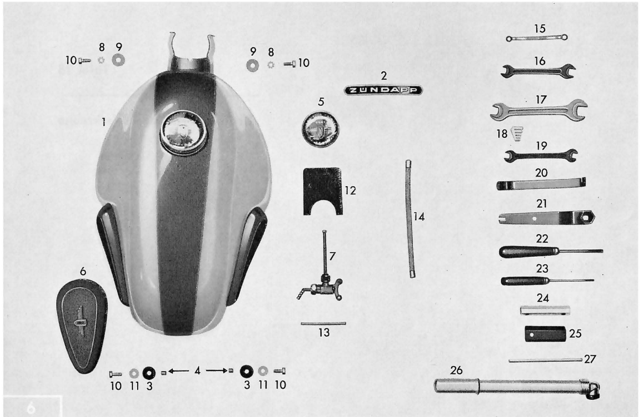
Tafel 15 Kraftstoffbehälter – Werkzeuge
