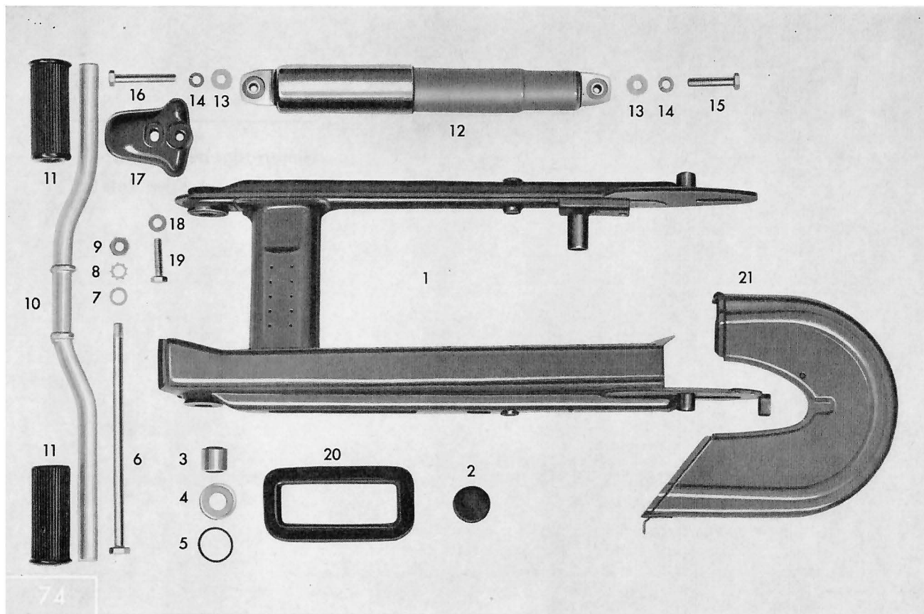
Tafel 4 a Hinterradgabel – Federbein
