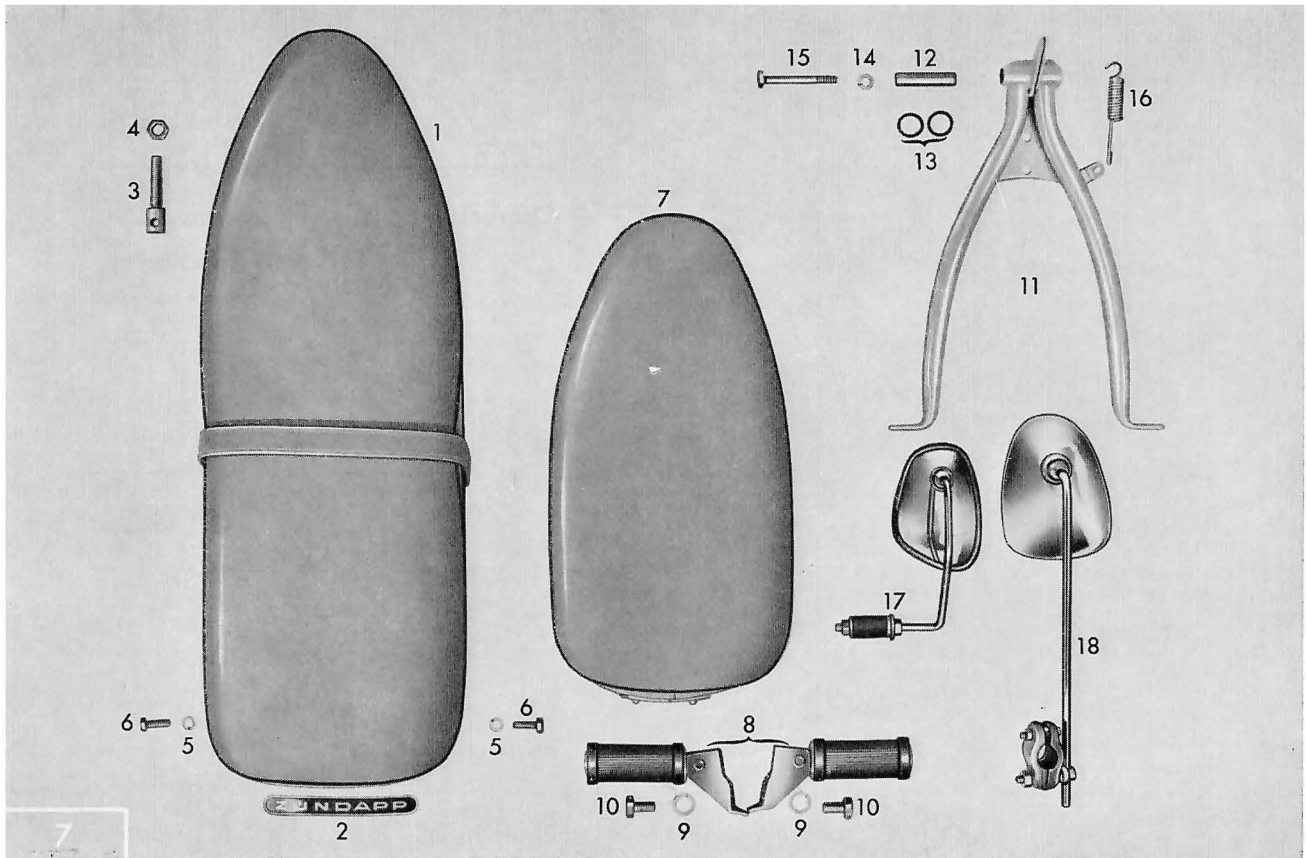
Tafel 16 a Doppelsitzbank – Einzelsitzbank – Radständer
