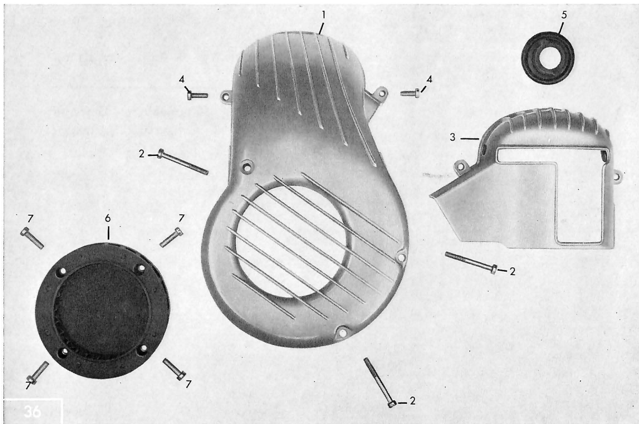
Tafel 3 a Lüftergehäuse – Lüfterrad
