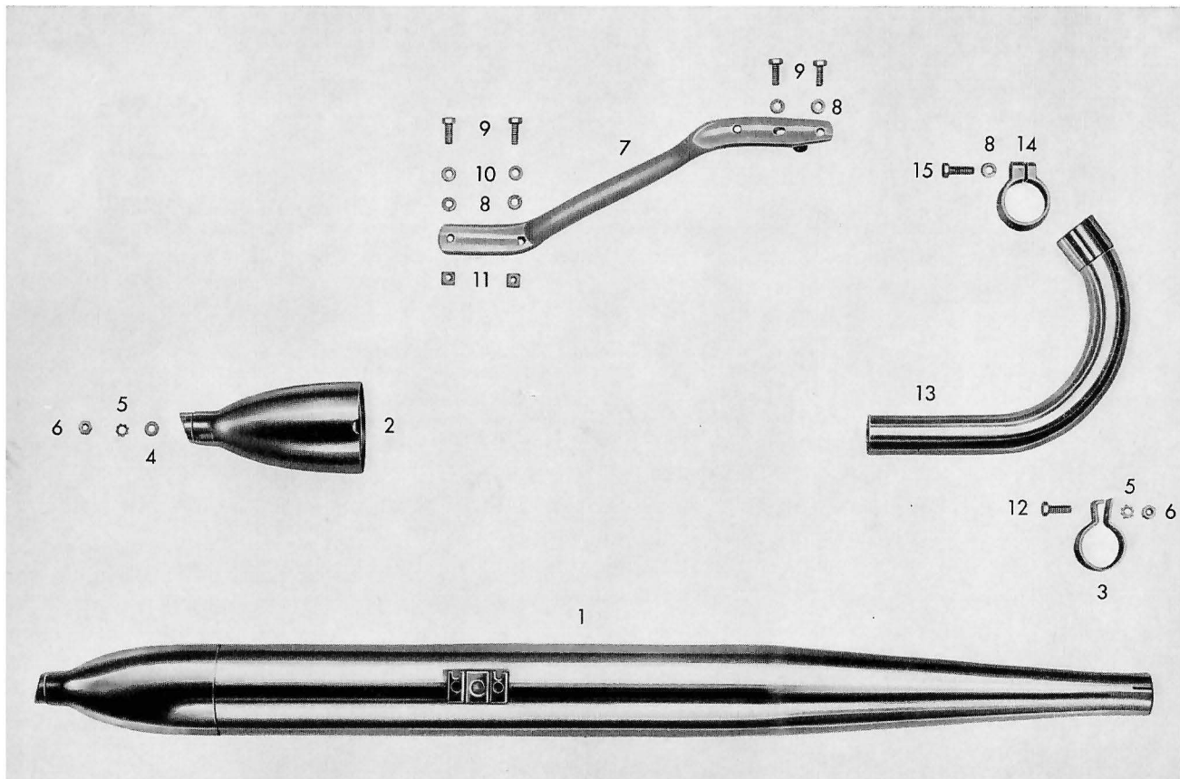
Tafel 13 α Auspuff
