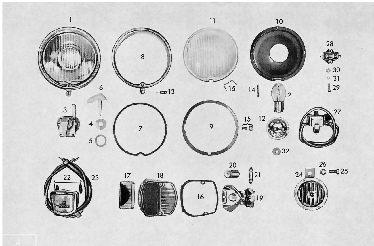
Tafel 10 Lichtanlage – Tachometer – Stopplicht (25 W Bilux)
