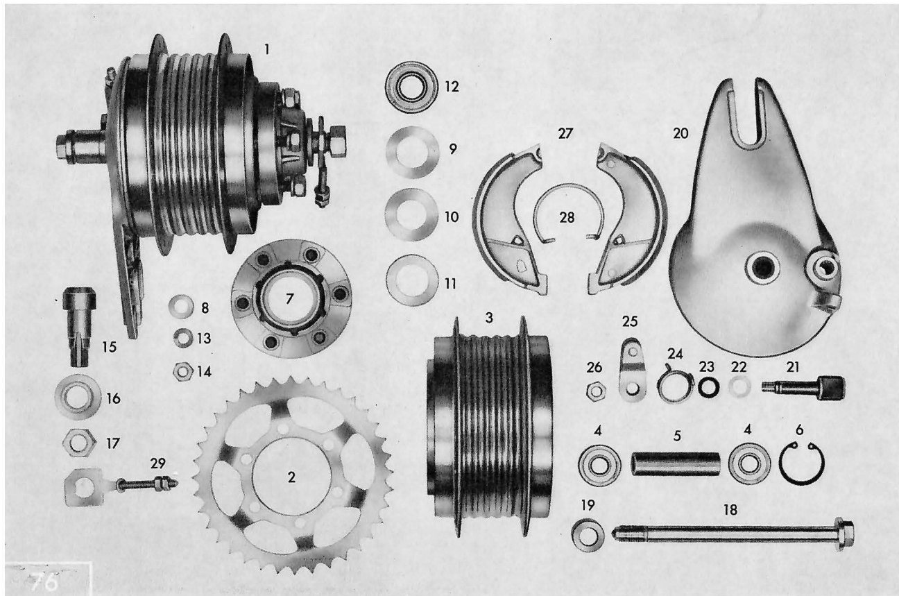
Tafel 8 a Hinteres Laufrad – Hinterradnabe 23" Räder
