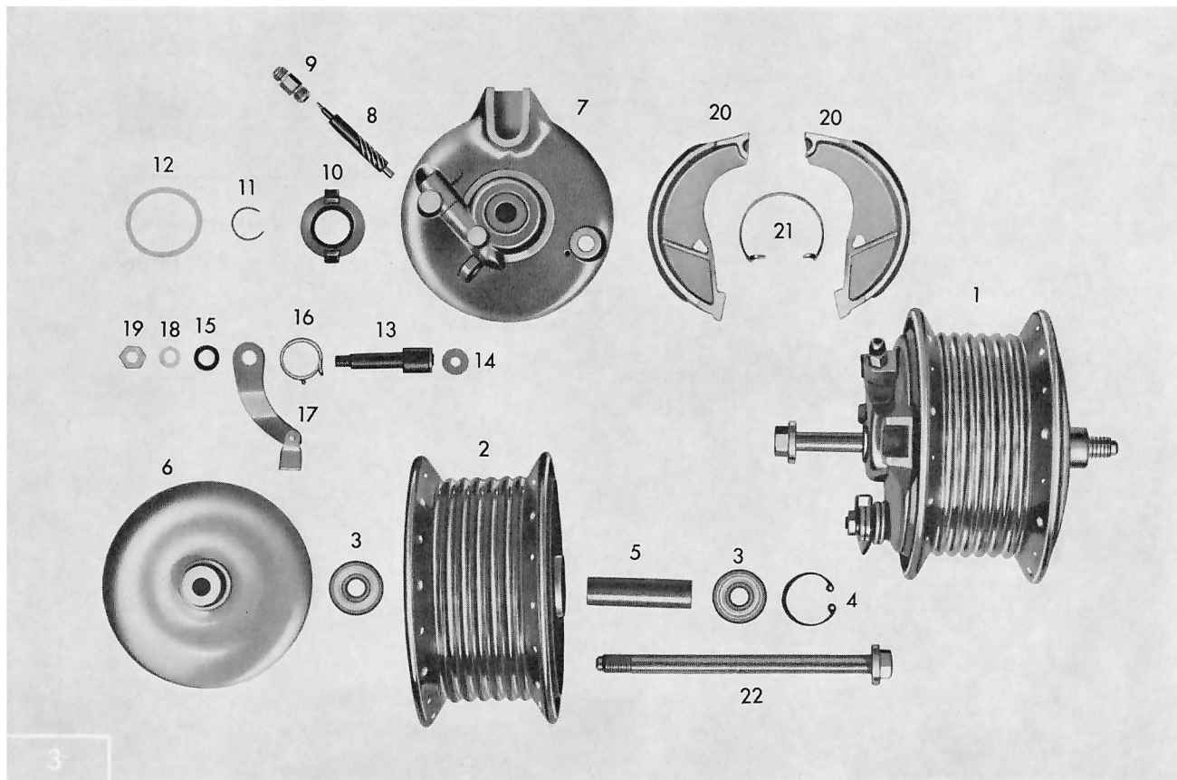
Tafel 6 Vorderes Laufrad – Vorderradnabe 23" Räder
