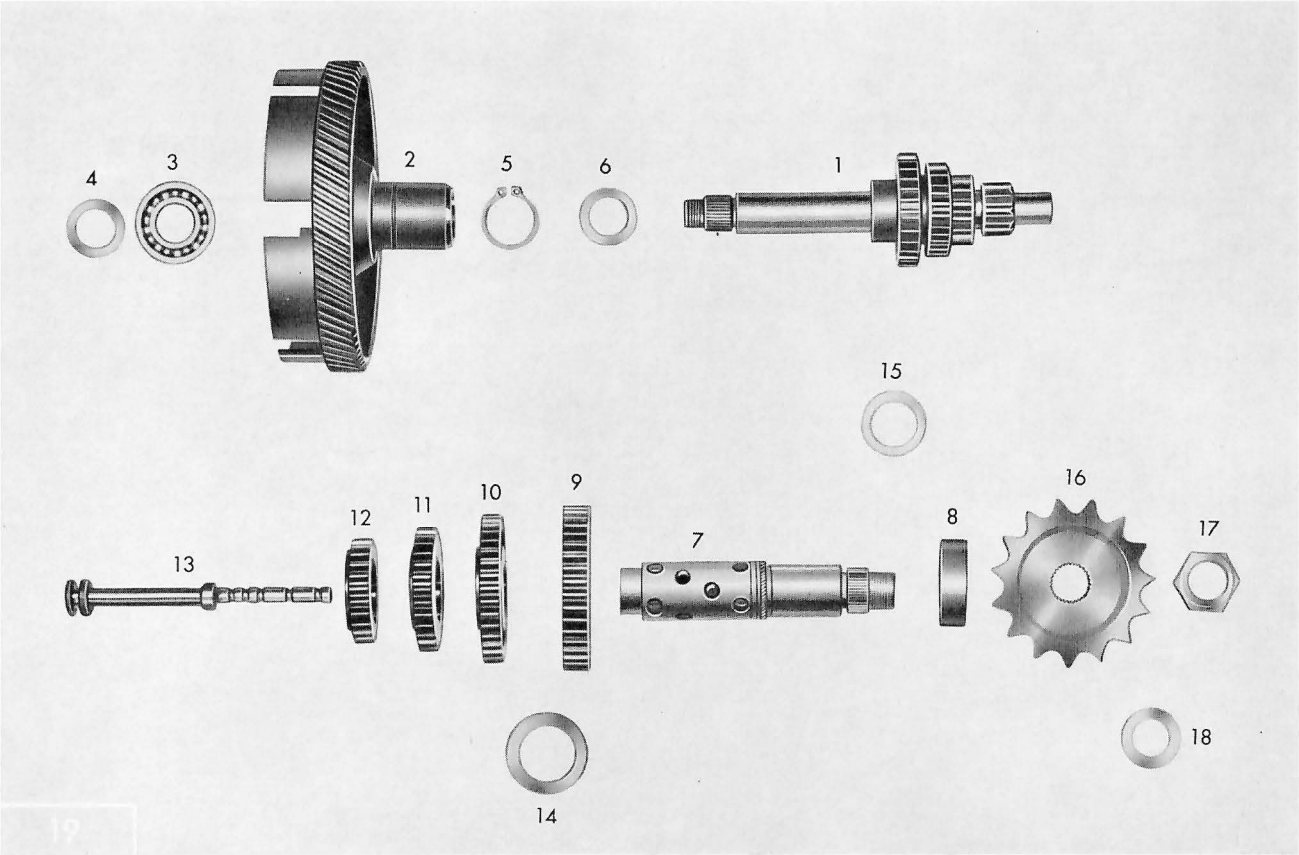
Tafel 8 Getriebe – Schaltwelle
