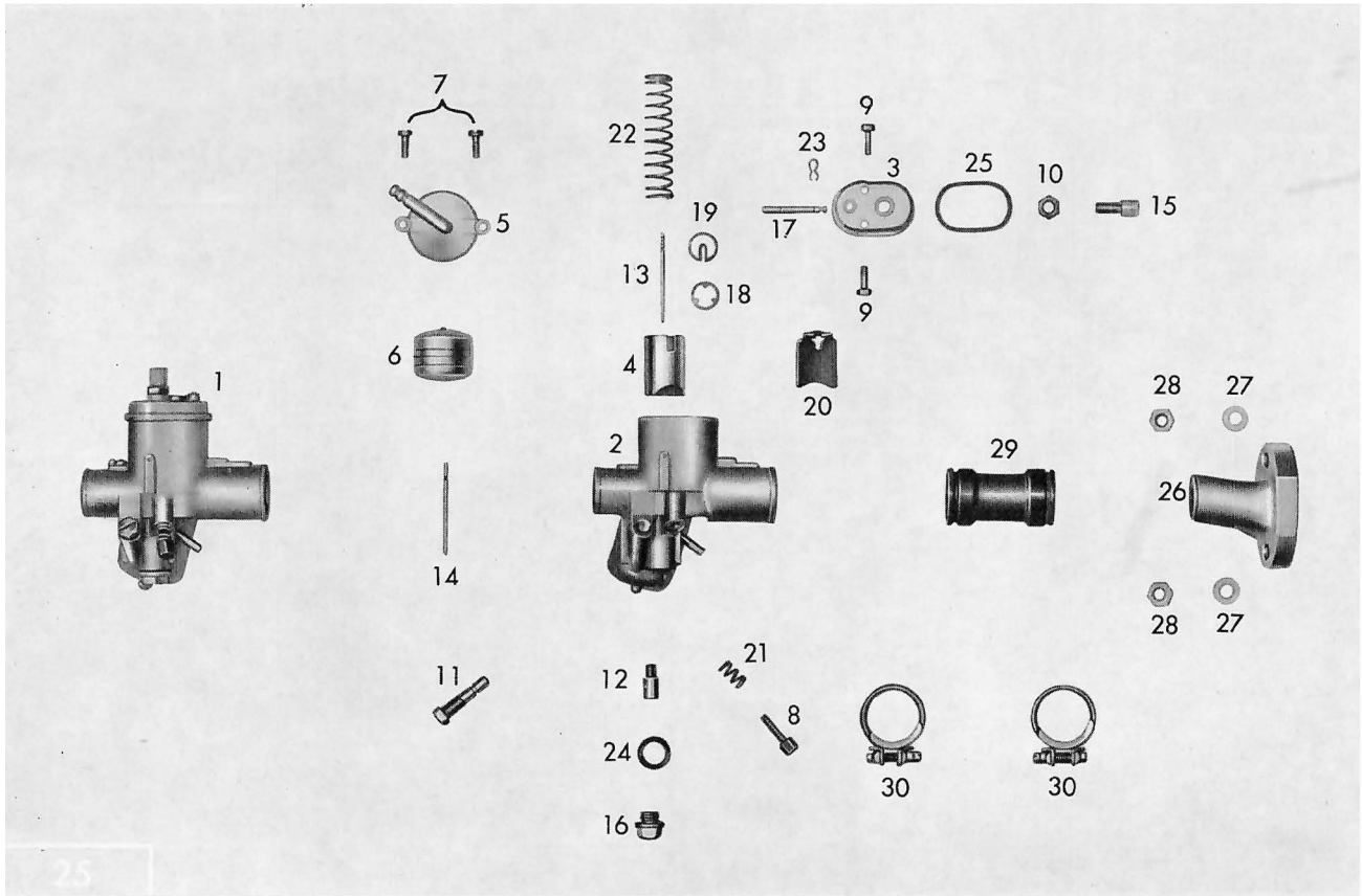
Tafel 7 Vergaser
