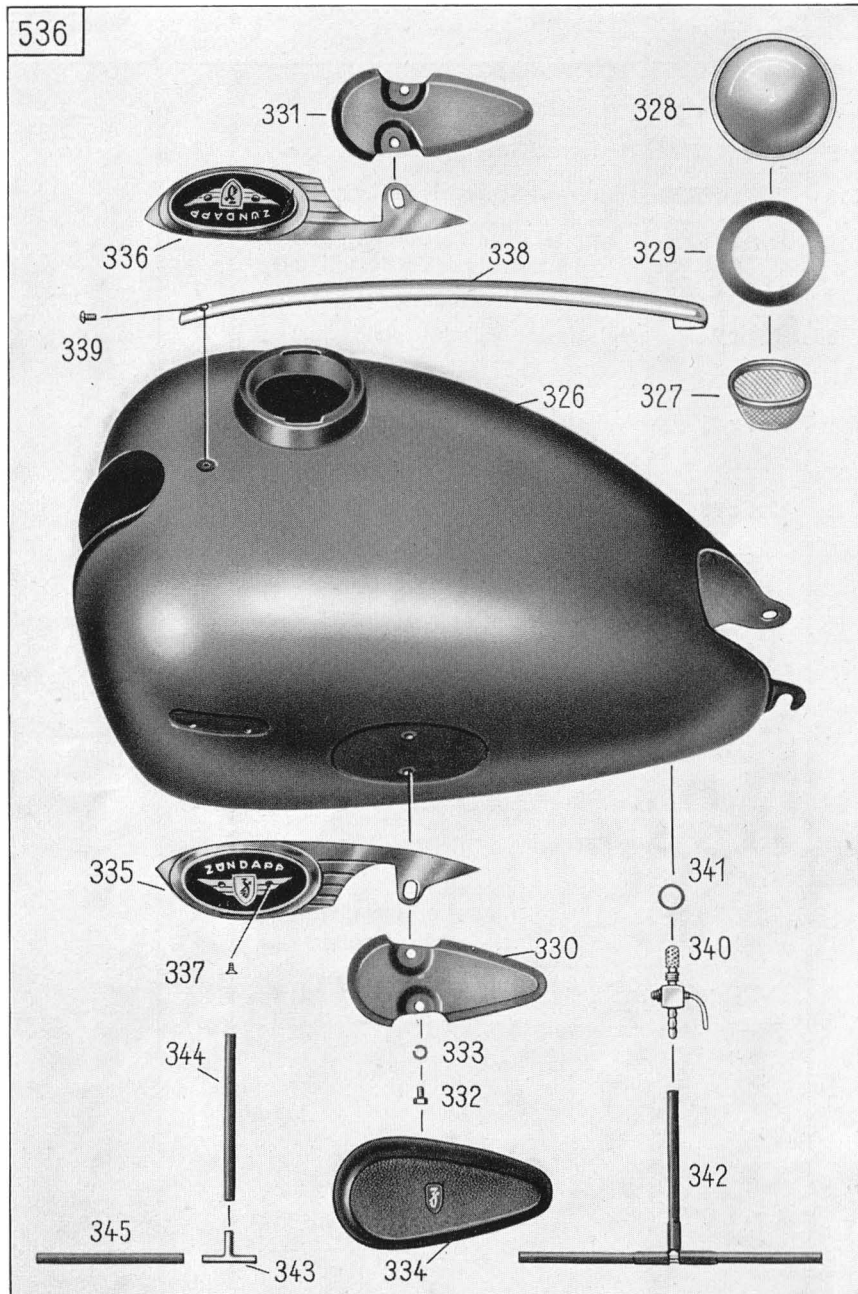
Tafel 18, Gruppe R: f) Kraftstoffbehälter und -leitungen
