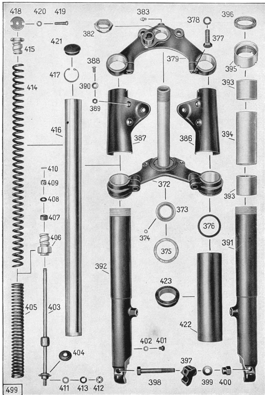
Tafel 20, Gruppe R: i) Federgabel, Zusammenbau Federgabelaufhängung
