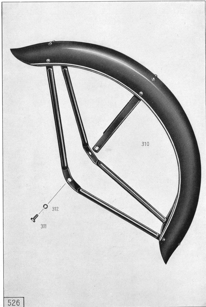
Tafel 16, Gruppe R: d) Schutzbleche, Vorderrad-Schutzblech
