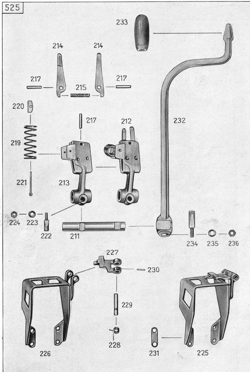
Tafel 10, Gruppe G: d) Fußschaltung
