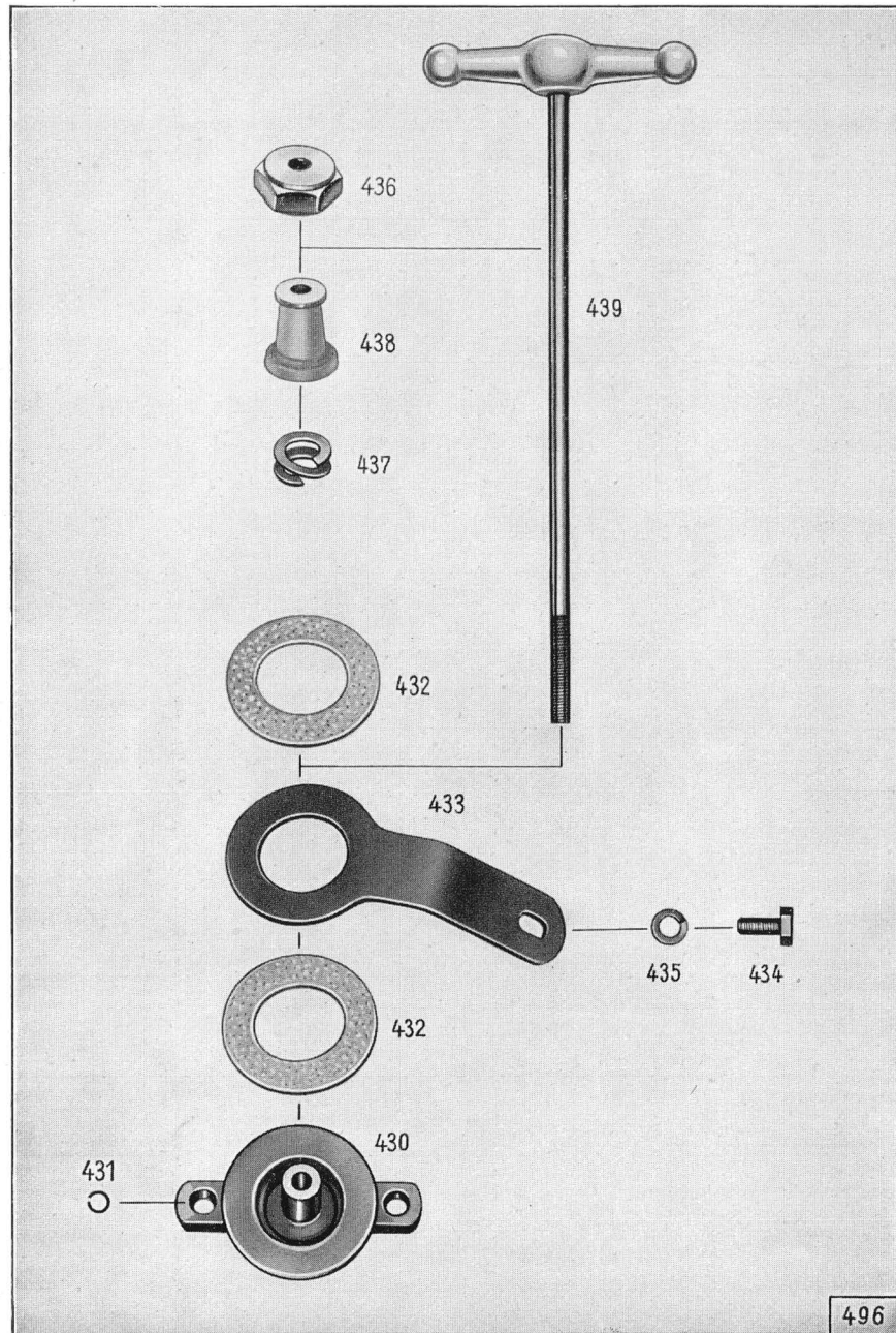
Tafel 21, Gruppe R: i) Federgabel, Steuerungsdämpfer
