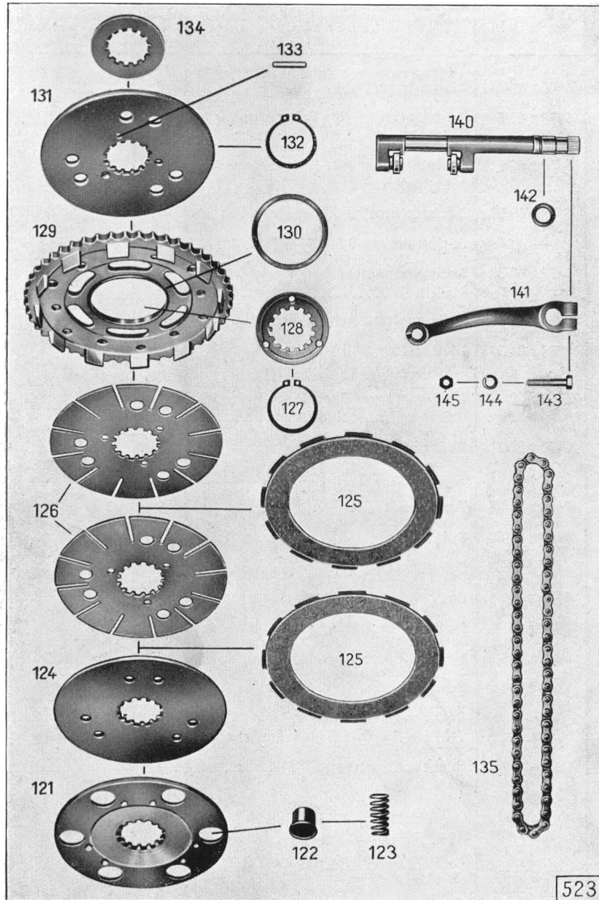
Tafel 7, Gruppe M: g) Kupplung, Kupplung, Kupplungsbetätigung
