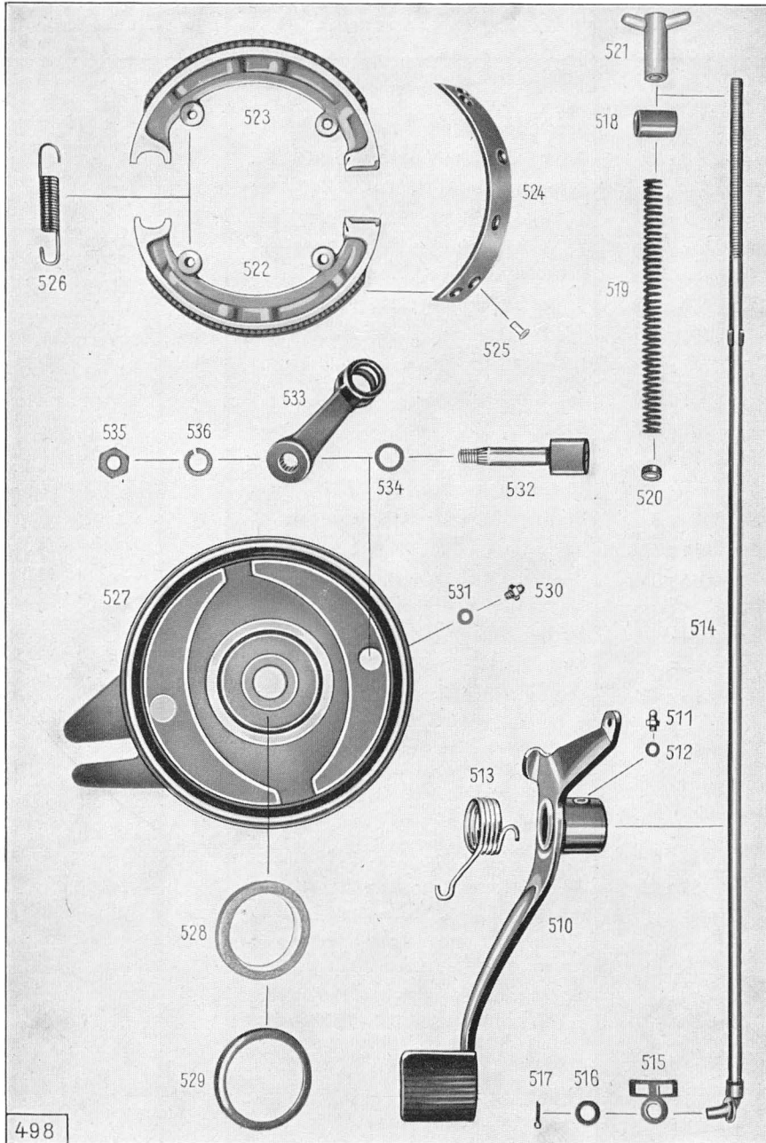
Tafel 24, Gruppe B: a) Bremsen, Fußbremse
