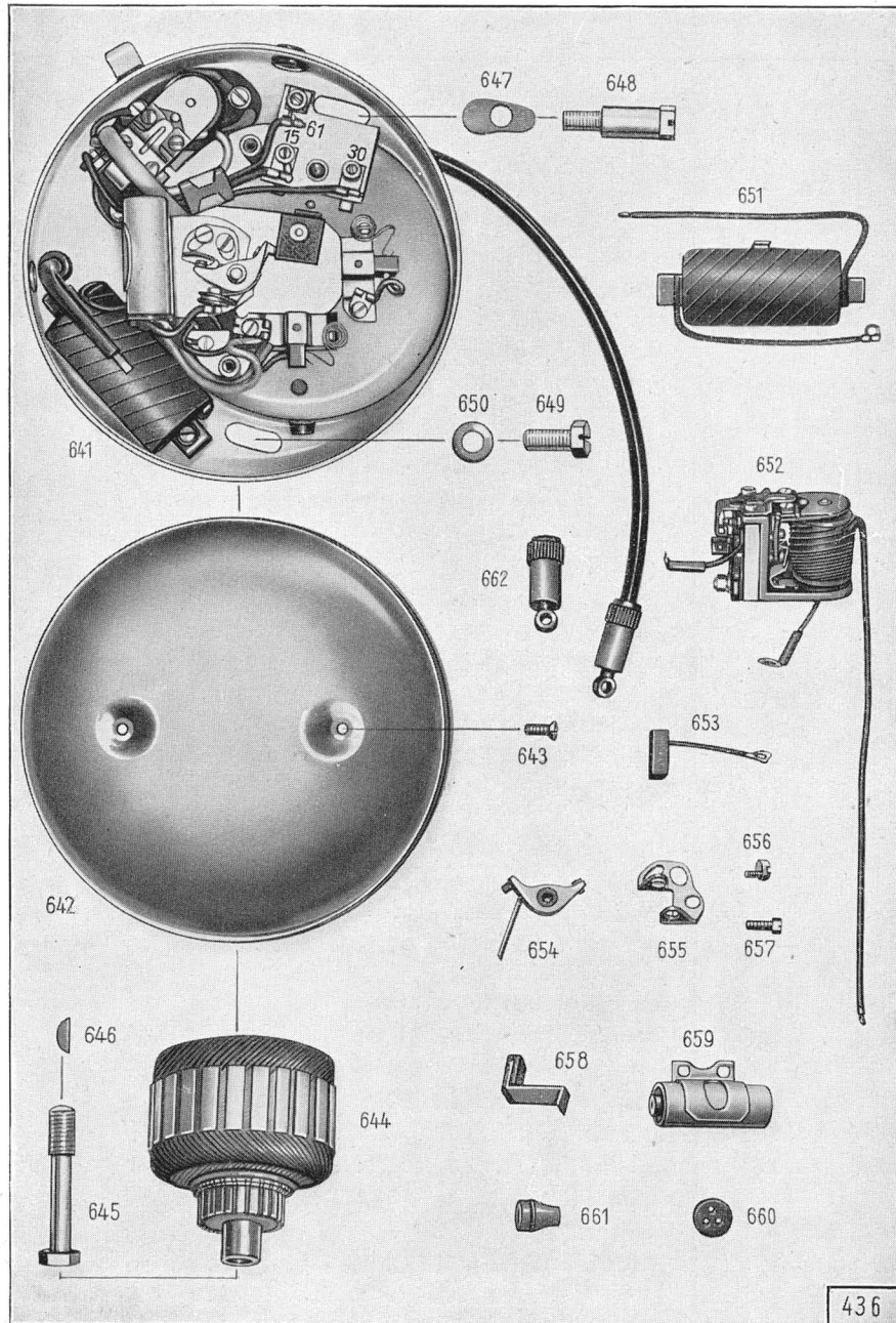
Tafel 28, Gruppe E: a) Elektrische Ausrüstung, Batterie-Lichtzünd-Anlage
