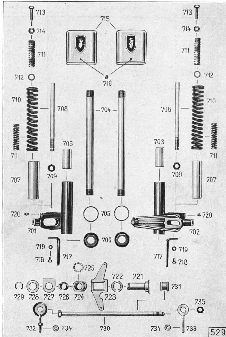
Tafel 13, Gruppe R: a) Rahmen
