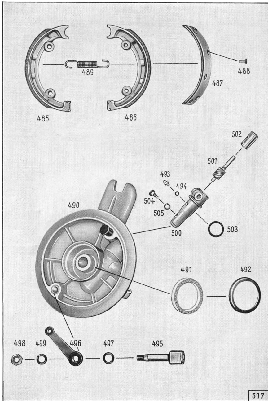
Tafel 23, Gruppe B: a) Bremsen Handbremse
