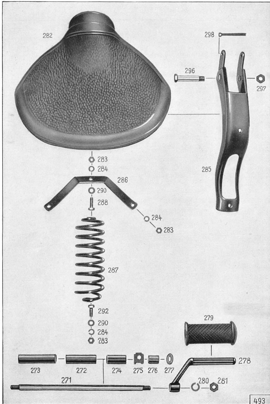
Tafel 14, Gruppe R: b) Fußraster und Sattel
