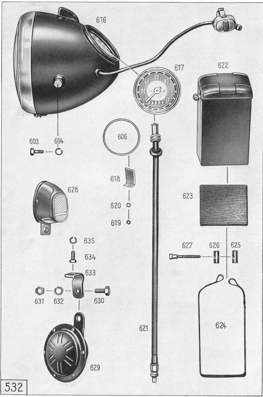
Tafel 27, Gruppe E: a) Elektrische Ausrüstung,
