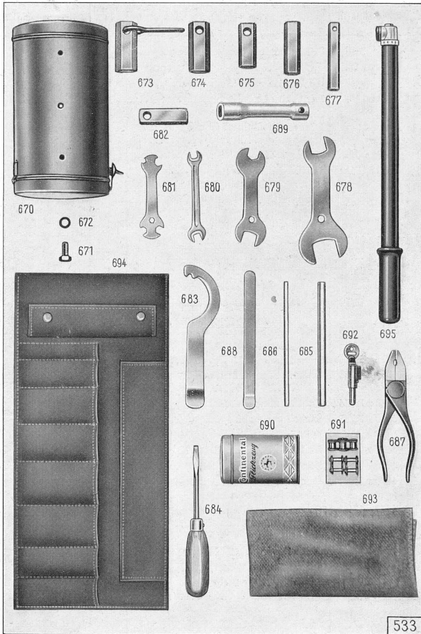
Tafel 29, Gruppe W: a) Werkzeug
