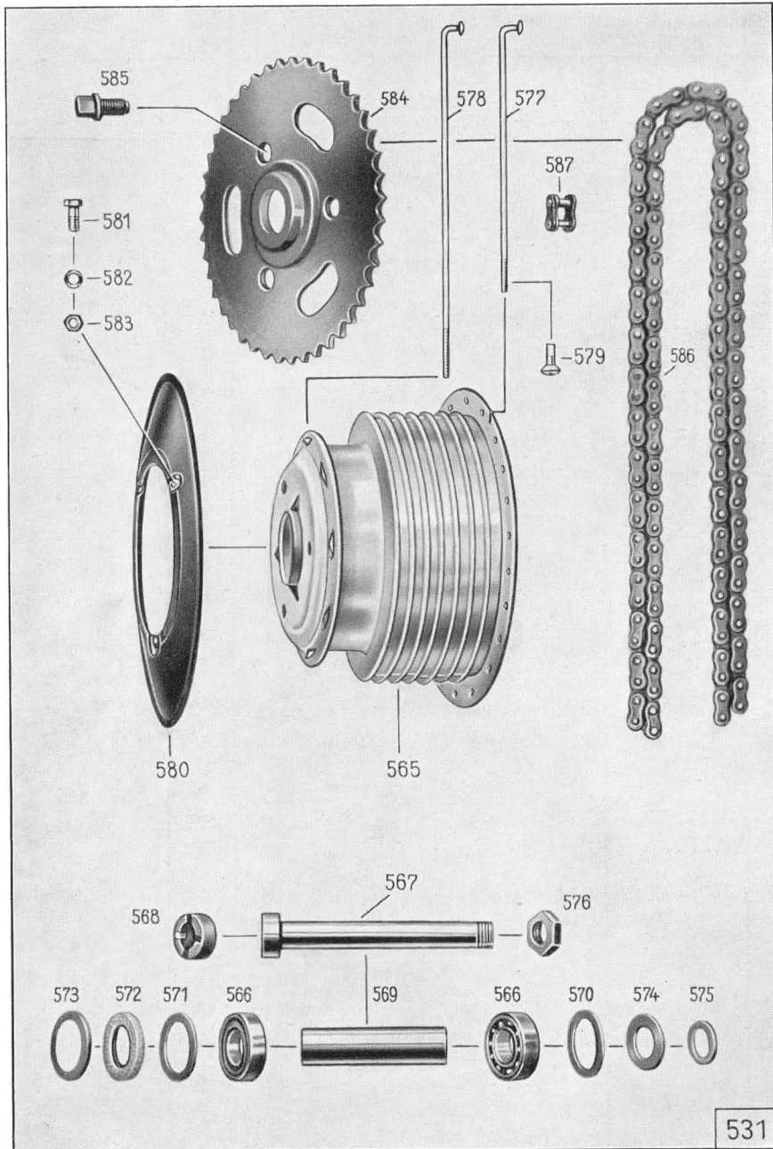
Tafel 26, Gruppe B: b) Räder, Hinterrad
