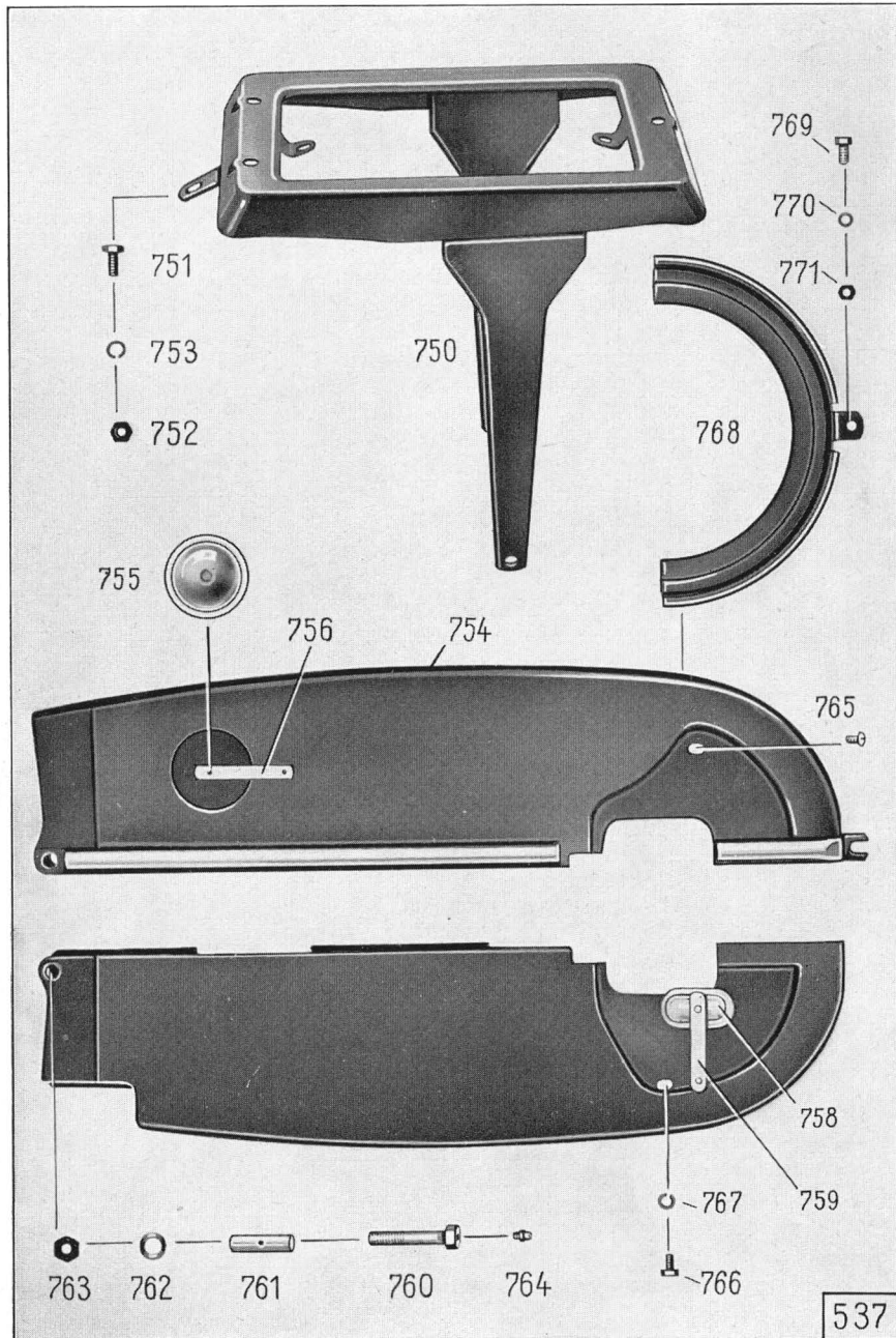
Tafel 15, Gruppe R: c) Gepäckträger und Kettenschutz
